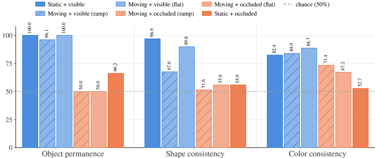
pairwise acc. (%)
