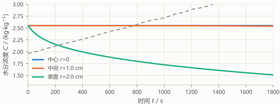
(b) 特征位置的水分浓度时程
