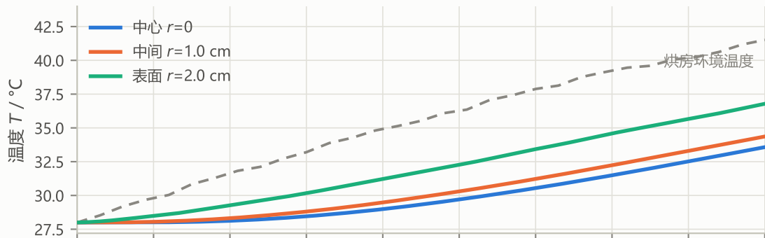
(a) 特征位置的温度时程
