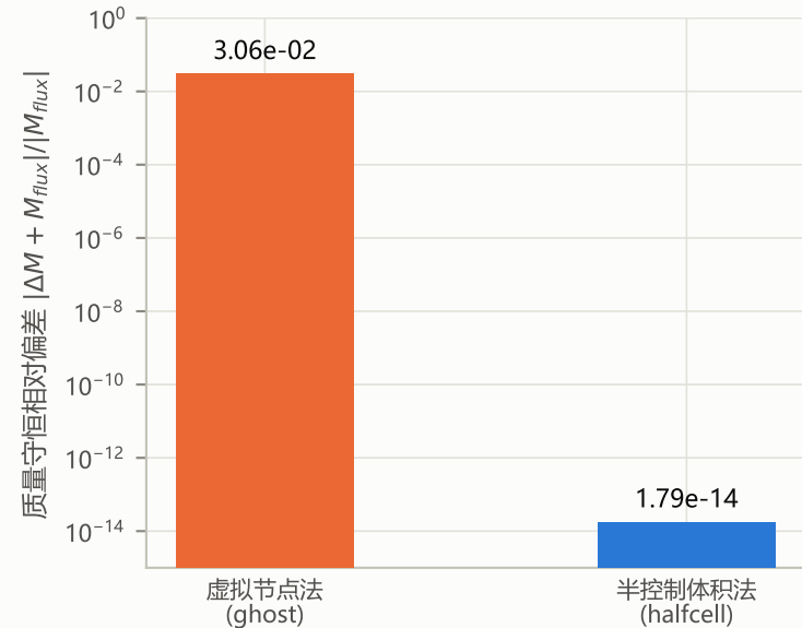
(a) 表面 Robin 离散的守恒性
