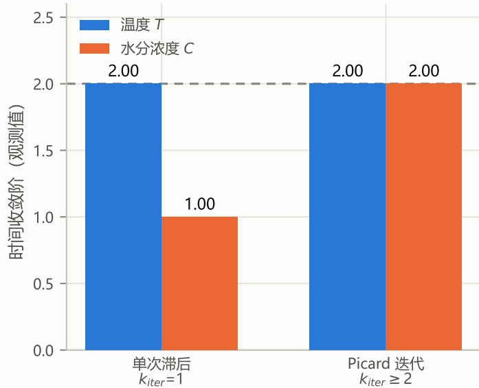
(b) D(C) 处理方式对时间精度的影响
