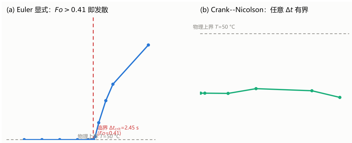
图 4: Euler 显式与 Crank–Nicolson 的稳定性对比: (a) 显式格式在 Fo > 0.41 后非物理发散 (对数刻度); (b) CN 格式任意 \Delta t 保持有界 (线性刻度)
