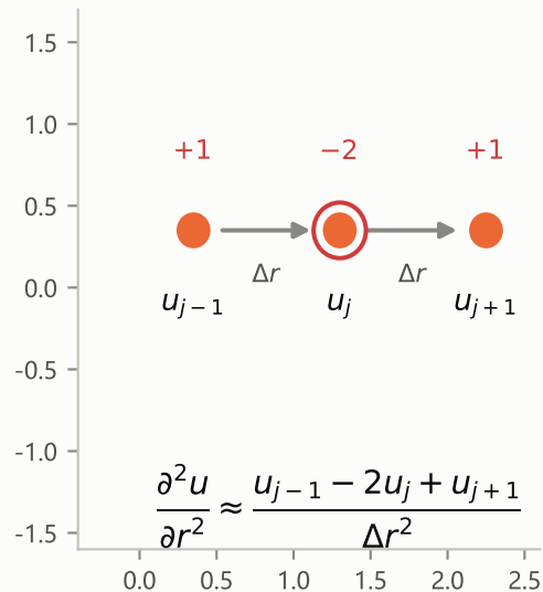
(b) 二阶中心差商 (空间 \partial^2 u / \partial r^2 )
