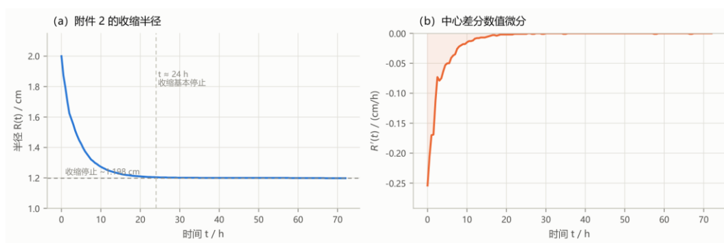
图 12 附件 2 收缩半径 R(t) 及其中心差分数值微分
