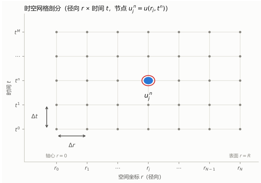
图 1 时空网格剖分 (径向 r \times 时间 t , 节点 u_j^n )
