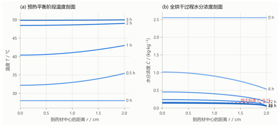
图 8 整个烘干过程的温度与水分浓度剖面
