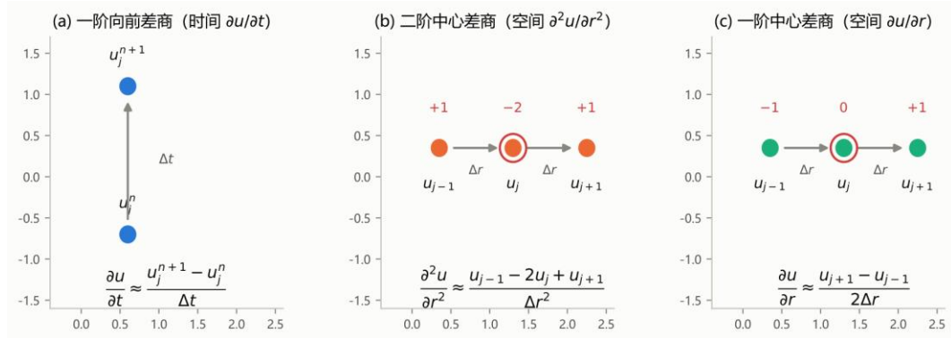
图 2 差商模板：(a) 一阶向前差商（时间）、(b) 二阶中心差商（空间）、(c) 一阶中心差商（空间）
