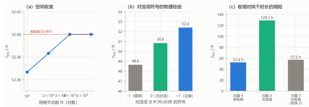
图 15 问题四的空间收敛、对流项符号检验与烘干时长对比
