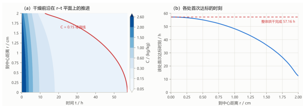
图 10 干燥前沿随时间的推进
