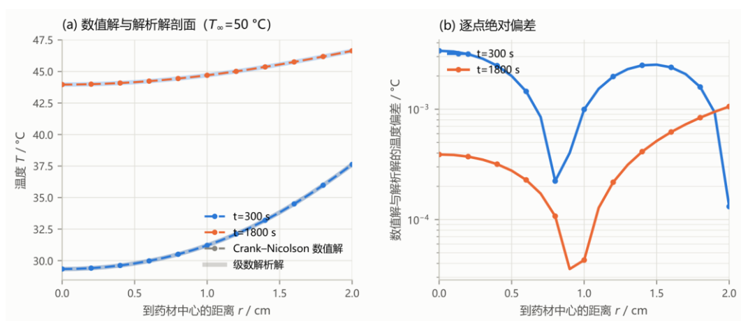
图 4 数值解与级数解析解对比（常环境纯导热）
