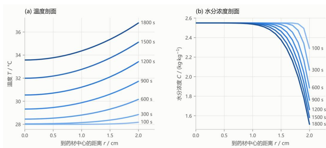
图 3 预热平衡阶段药材温度与水分浓度剖面
