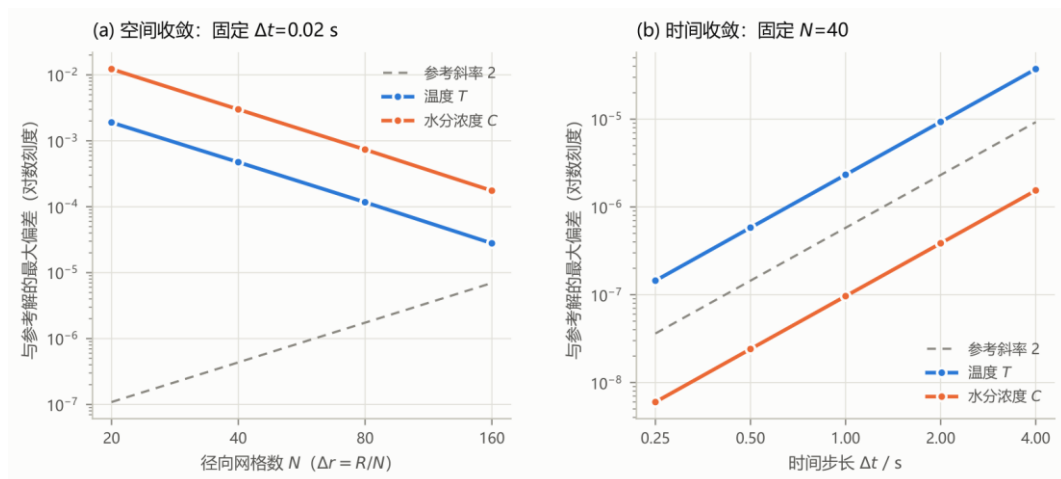
图 5 空间与时间方向的收敛阶验证
