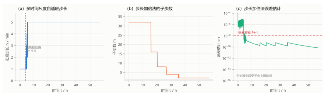
图 11 自适应时间步长与误差控制
