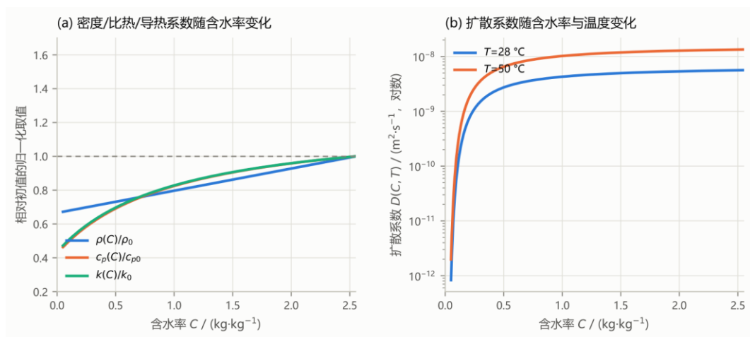
图 7 附录 3 变参数物性随水分浓度的变化
