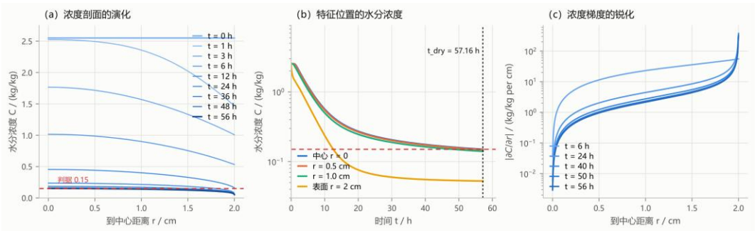
图 9 烘干全过程的水分浓度剖面与特征位置时程
