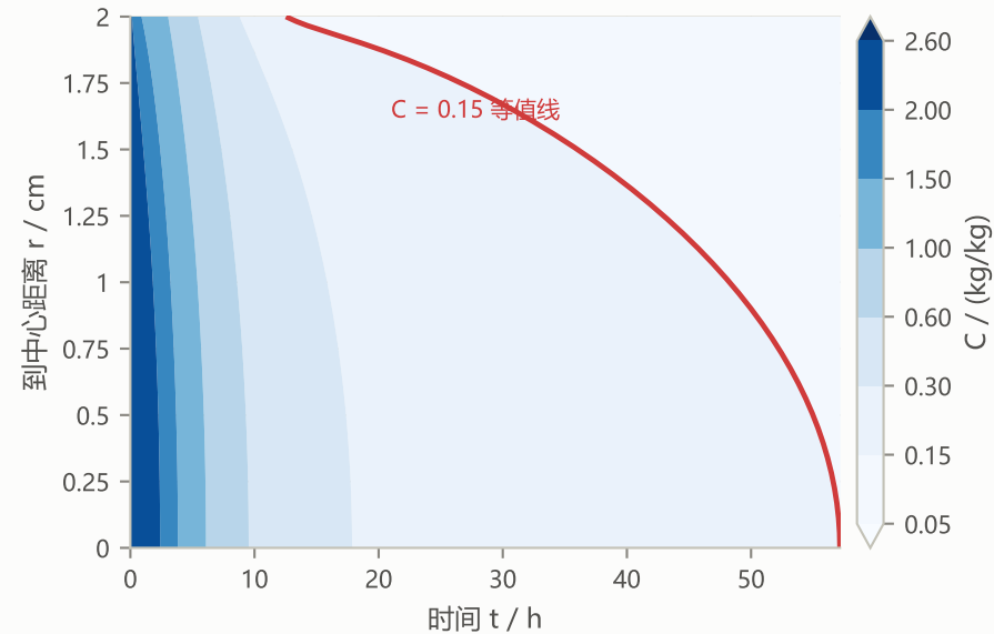
(a) 干燥前沿在 r - t 平面上的推进
