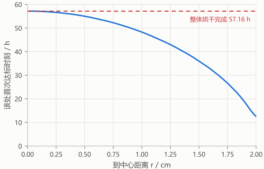
(b) 各处首次达标的时刻
