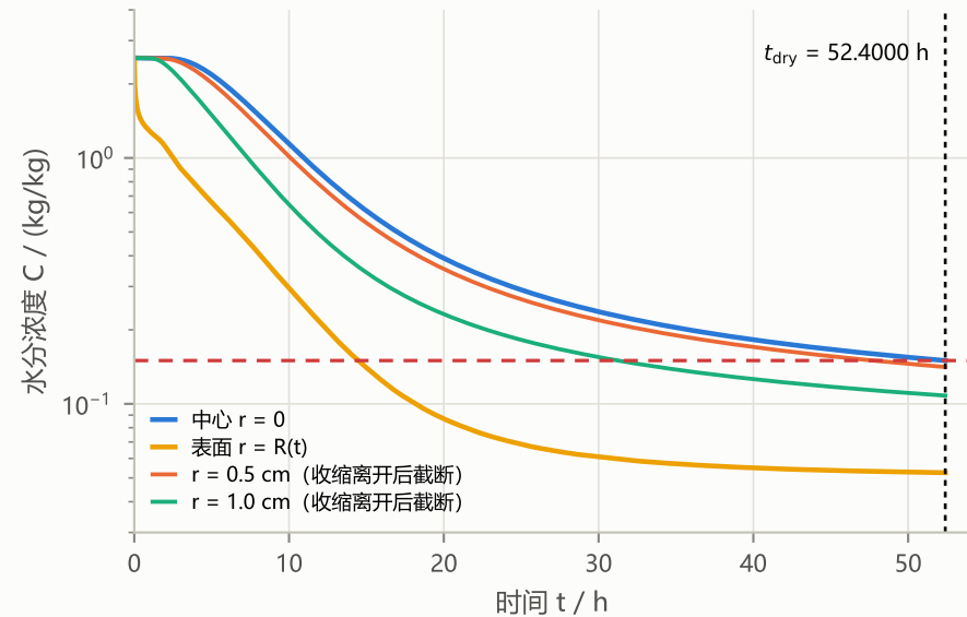
(a) 特征位置的水分浓度
