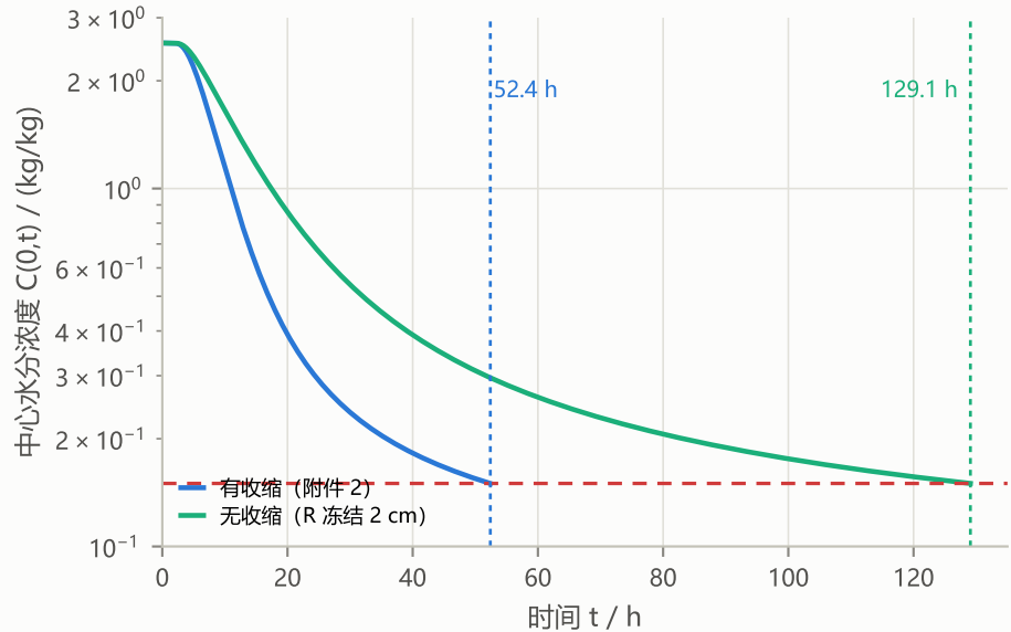
(b) 收缩显著缩短烘干时长
