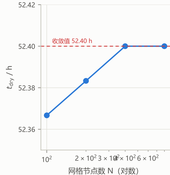
(a) 空间收敛
