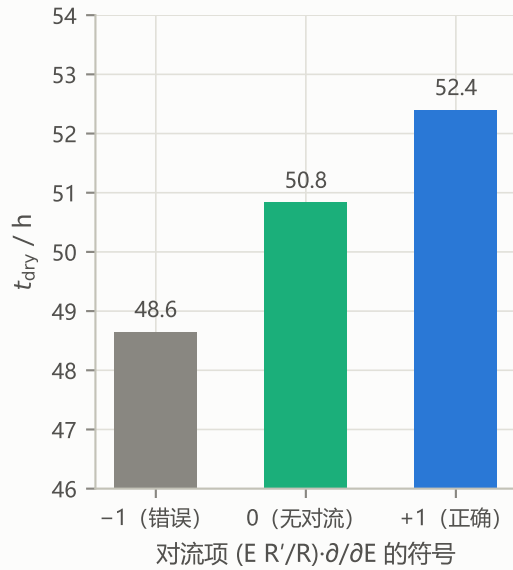
(b) 对流项符号的物理检验
