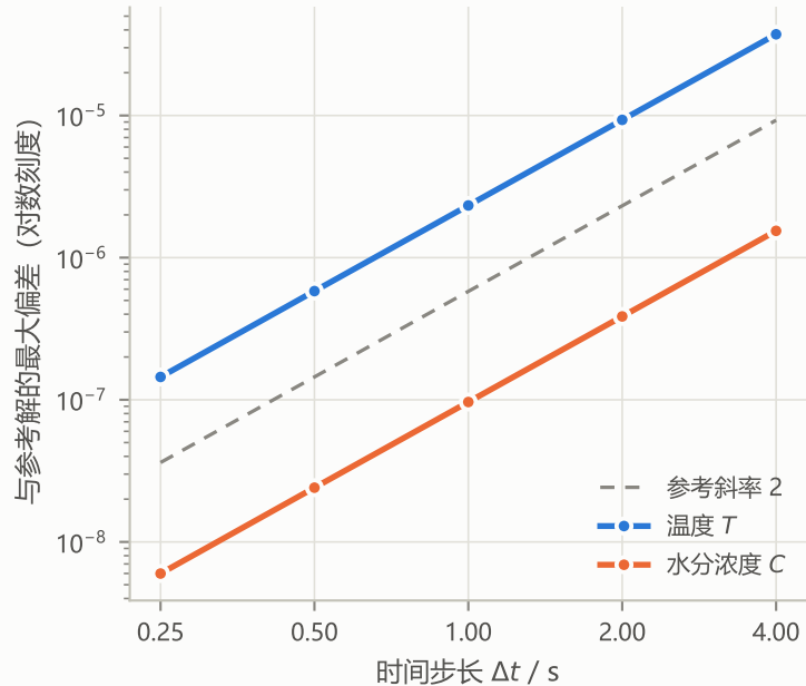
(b) 时间收敛: 固定 N=40
