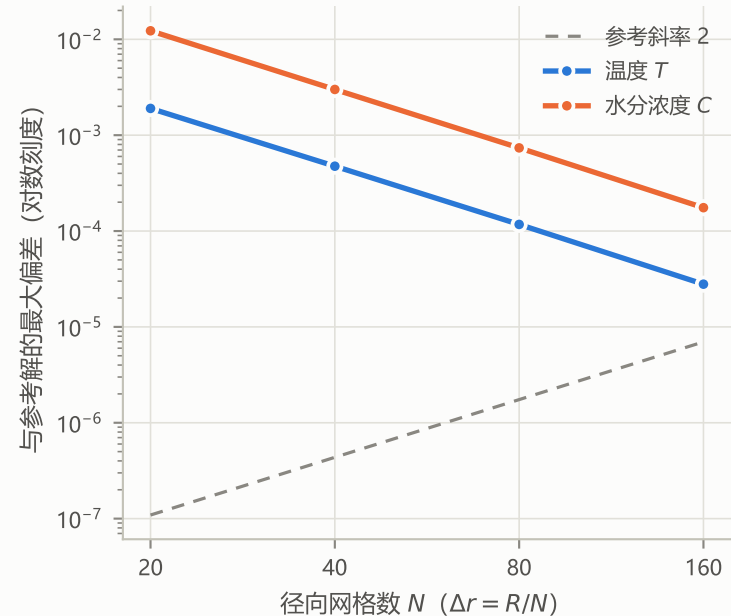
(a) 空间收敛: 固定 \Delta t=0.02 s
