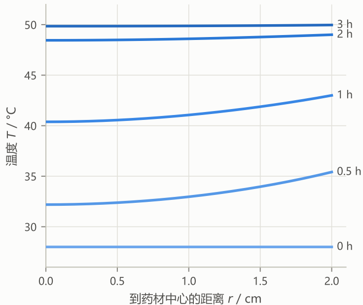
(a) 预热平衡阶段温度剖面
