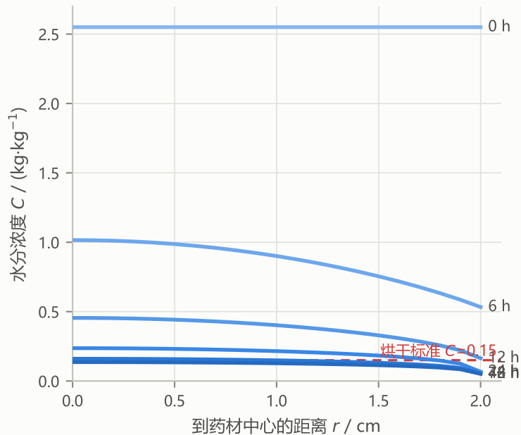
(b) 全烘干过程水分浓度剖面
