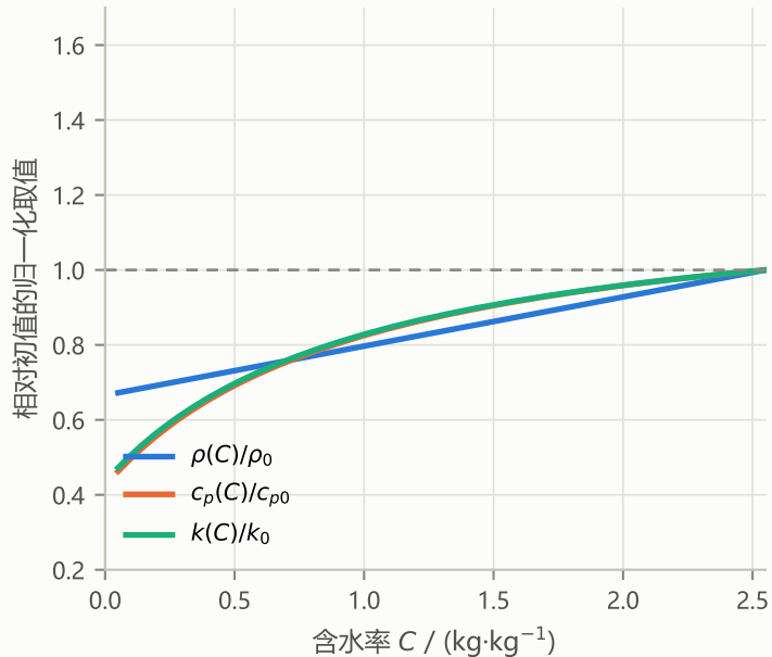
(a) 密度/比热/导热系数随含水率变化
