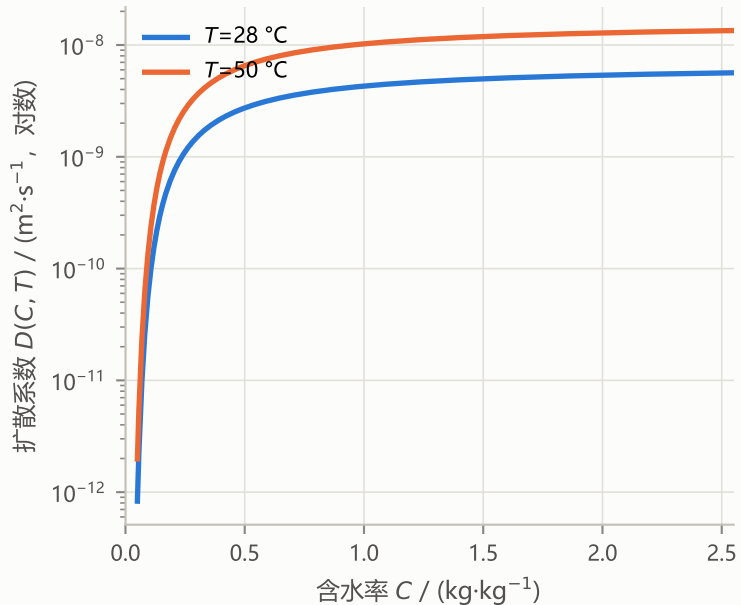
(b) 扩散系数随含水率与温度变化
