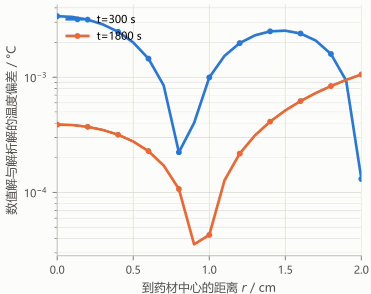
(b) 逐点绝对偏差
