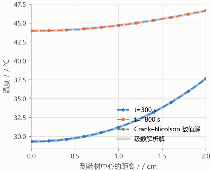
(a) 数值解与解析解剖面 ( T_{\infty}=50\text{ }^{\circ}\text{C} )
