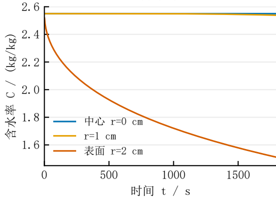
(b) 含水率时程
