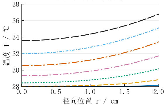
(a) 中截面温度分布
