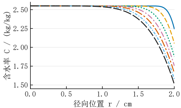
(b) 中截面含水率分布
