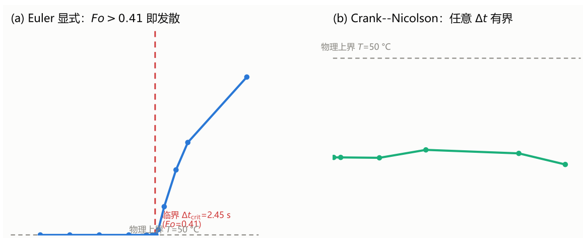
图 7: Euler 显式与 Crank–Nicolson 的稳定性对比: (a) 显式格式在 Fo > 0.41 后非物理发散 (对数刻度); (b) CN 格式任意 \Delta t 保持有界 (线性刻度)
