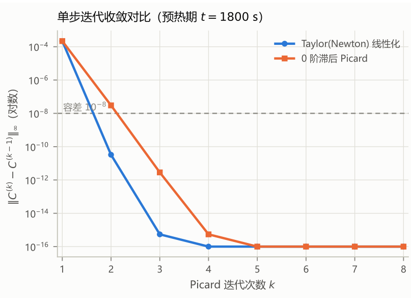
图 5: Taylor(Newton) 线性化与 0 阶滞后 Picard 的单步迭代收敛对比
