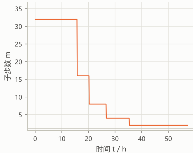
(b) 步长加倍法的子步数
