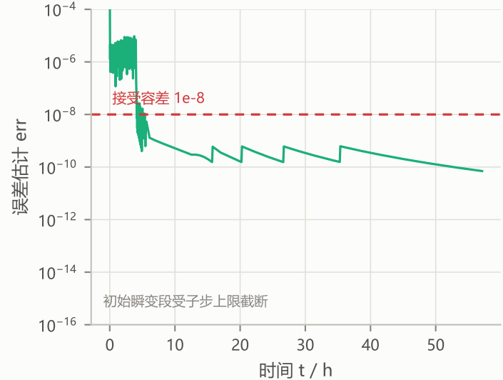
(c) 步长加倍法误差估计
