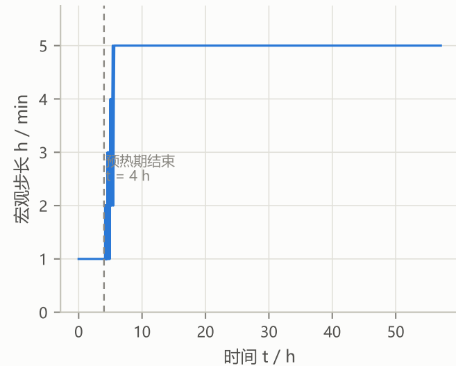
(a) 多时间尺度自适应步长
