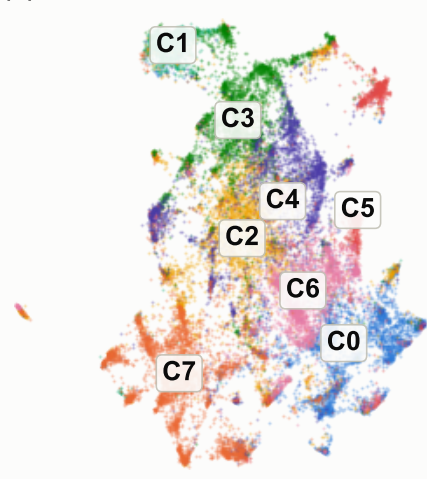
(b) UMAP
