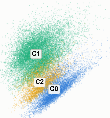
(a) PCA
