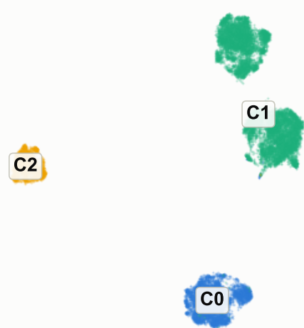
(b) UMAP
