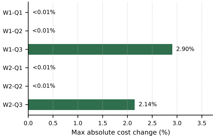
Cost robustness across eta
