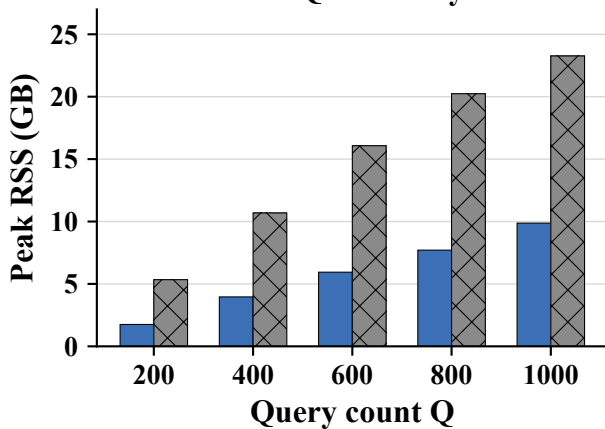
W2-Q1 Memory
