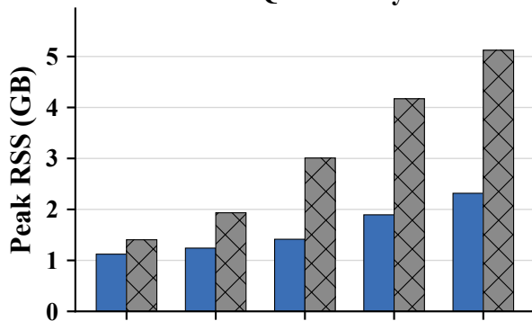
W2-Q1 Memory
