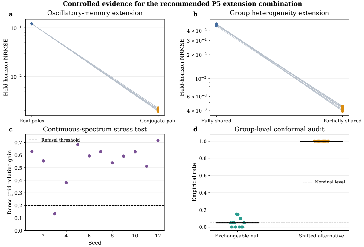
图 7: 受控扩展审计。(a) 阻尼振荡上正实极点与共轭极点对外推比较。(b) 组间异质条件下完全共享与部分共享衰减率的比较。(c) 稠密谱相对三阶有限模型的改善, 虚线为声明的模型失配阈值。(d) 组级 conformal 的误报率和偏移备择检出率。各面板只在同一受控任务内部比较方法。
