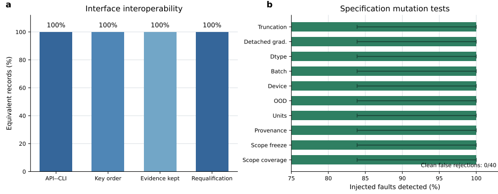
Figure 2: 参考实验验证。(a) API-命令行等价性、键顺序不变性、迁移证据保留及强制重新判定, 各 40 轮; (b) 10 类规范变异, 每类 20 轮, 误差线为 Wilson 95% 区间。有效记录误拒为 0/40。
