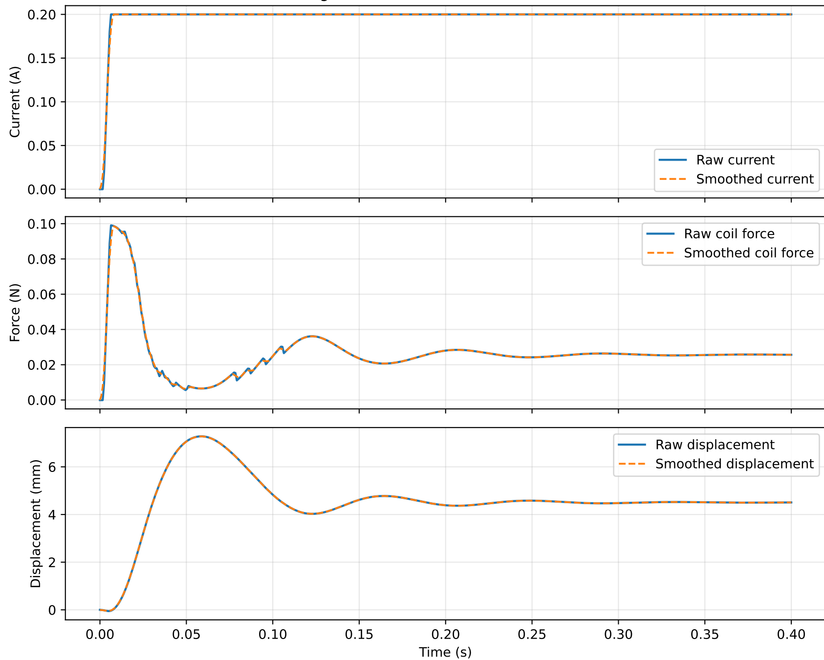
Single Actuator ESA Dataset Overview
