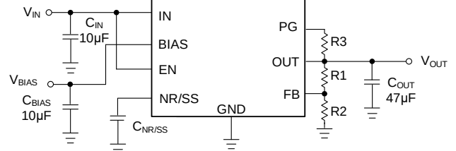
图 2 GM1203-2 典型应用
