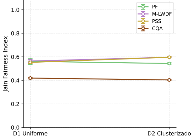
Figura 7: Jain bajo T2: M-LWDF y PSS mejoran con D2; PF empeora. Las líneas se cruzan.
