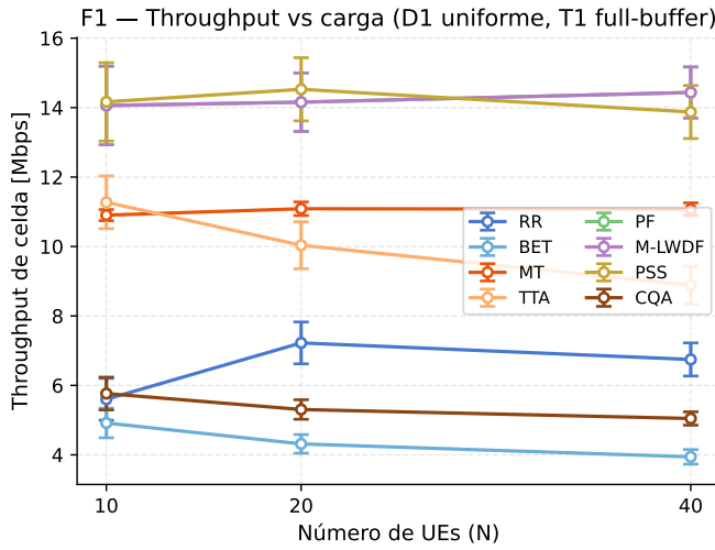
Figura 1: Throughput de celda vs N (D1, T1). PF sube de forma estable; PSS alcanza su máximo en N=20 y baja en N=40; BET cae porque dedica más tiempo a UEs de canal débil.
