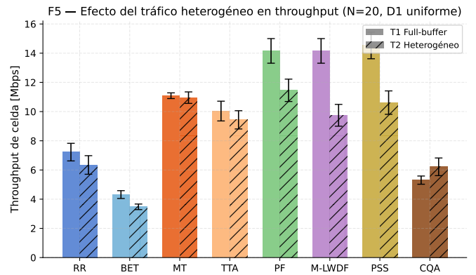
Figura 5: Throughput total: T1 vs T2 (N=20, D1). La paradoja: M-LWDF cae más que cualquier otro.
