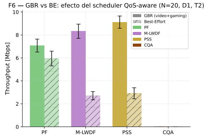
Figura 6: Throughput GBR vs BE bajo T2. M-LWDF favorece GBR; PF no distingue entre tipos.
