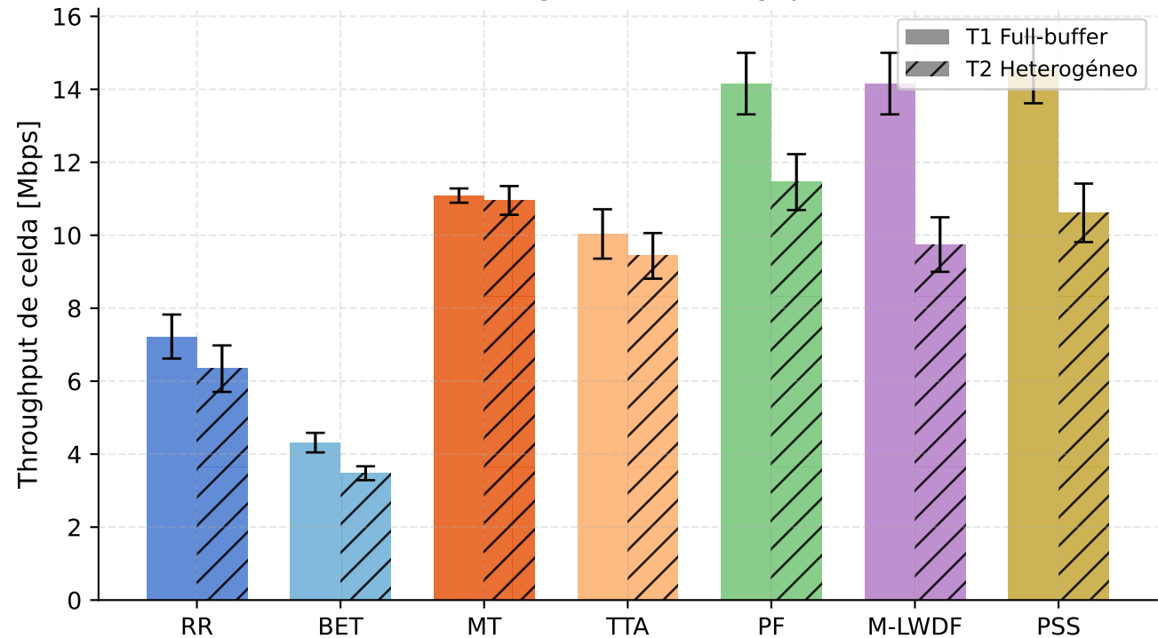
F5 — Efecto del tráfico heterogéneo en throughput (N=20, D1 uniforme)
