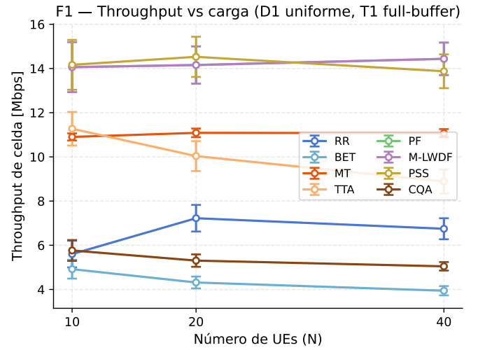
Figura 1: Throughput de celda vs N (D1, T1). PSS y PF escalan bien; BET penaliza por equidad.
