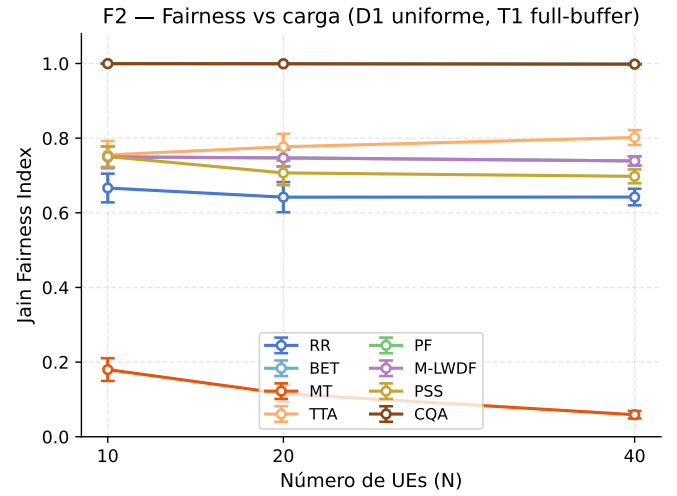
Figura 2: Jain vs N (D1, T1). MT colapsa con N; TTA y PF son estables.
