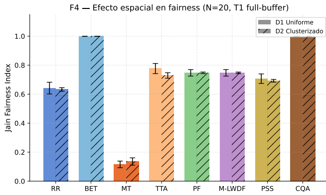
Figura 4: Jain D1 vs D2, N=20, T1. MT tiene fairness mala en ambas condiciones.
