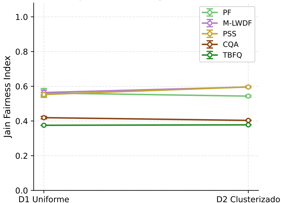
F8 — Fairness bajo tráfico heterogéneo: D1 vs D2 (N=20, T2)
