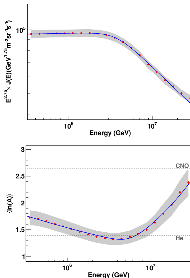
図 1.5 LHAASO-KM2A が測定した全粒子エネルギースペクトル（上）と \langle \ln A \rangle （下）。灰色帯は系統的な不確かさ、青線は折れ曲がりを含む適合結果を表す。LHAASO Collaboration (2024) の Fig. 3 より引用 [13]。
