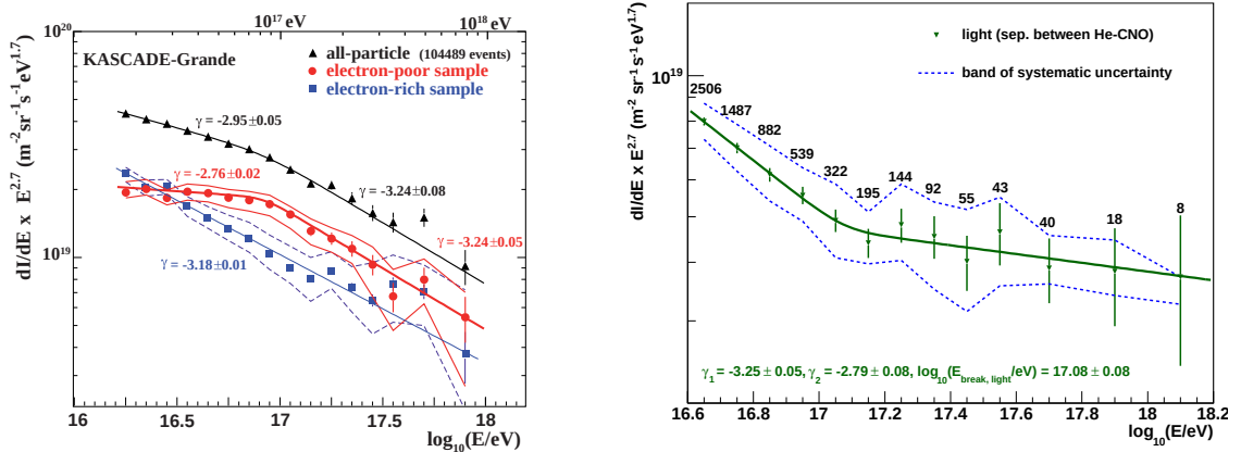
図 1.8 KASCADE-Grande が再構成した質量群別エネルギースペクトル。左は全粒子、電子成分の少ない試料、電子成分の多い試料の比較であり、電子成分の少ない試料は約 8 \times 10^{16} eV で急峻化する。右では、電子成分の多い試料のスペクトルの傾きが約 10^{17.08} eV から緩やかになる。左は KASCADE-Grande Collaboration (2011) の Fig. 4、右は同 Collaboration (2013) の Fig. 5 より引用 [45, 49]。
