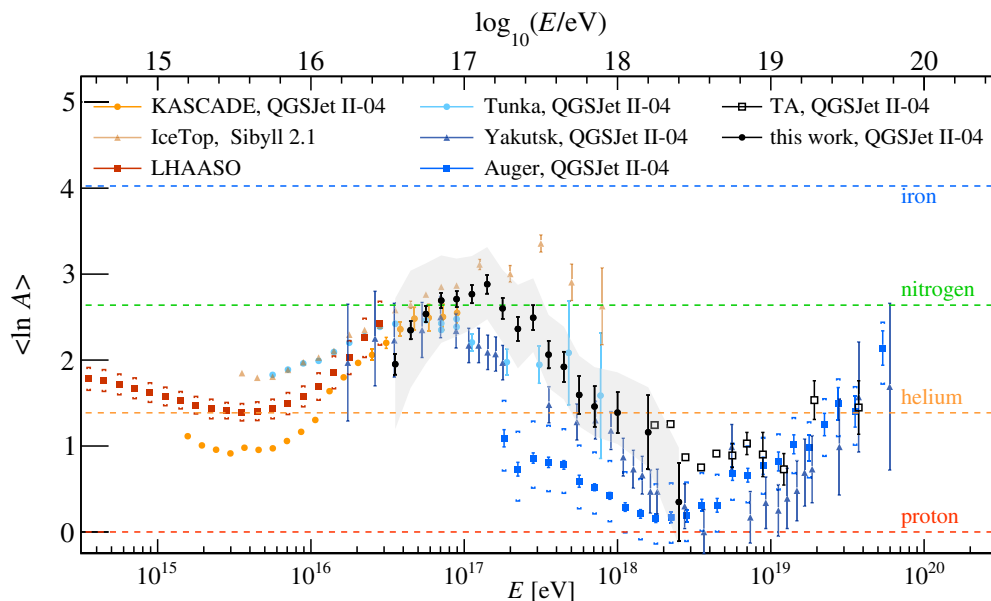
図 1.3 宇宙線の \langle \ln A \rangle 。TALE ハイブリッド質量組成測定の Fig. 22 より引用 [21]。
