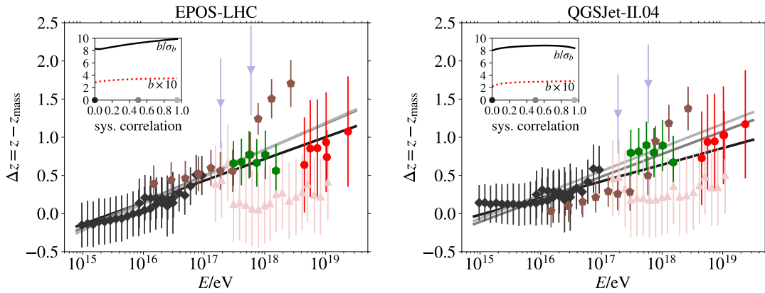
図 2.2 8 つの空気シャワー実験によるミュオン測定を共通尺度で比較したメタ解析。縦軸は質量組成の期待値を差し引いた \Delta z = z - z_{\max} 、横軸は一次エネルギーである。左は EPOS-LHC、右は QGSJetII-04 に対する比較を示す。直線は実験内の系統的な不確かさの相関を変えた適合であり、KASCADE-Grande と EAS-MSU の点はエネルギースケールを相互較正していない。Dembinski et al. (2019) の Fig. 10 より引用 [69]。
