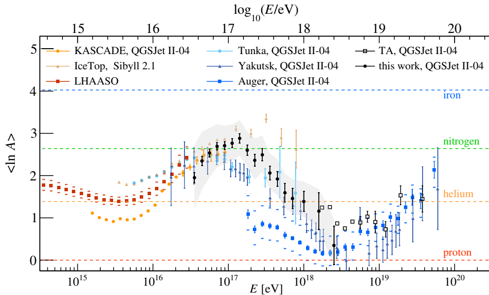
図 1.5 宇宙線の平均対数質量 \langle \ln A \rangle 。TALE ハイブリッド質量組成測定 Fig. 22 より引用 [44]。
