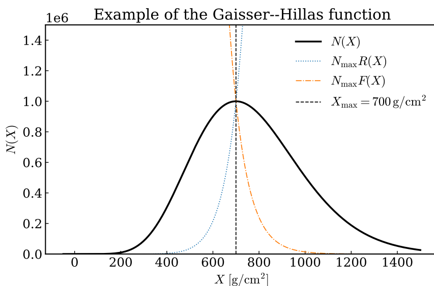
図 1.7 Gaisser–Hillas 関数の例。 N_{\max} = 10^6 、 X_{\max} = 700 \text{ g/cm}^2 、 X_0^{\text{GH}} = -50 \text{ g/cm}^2 、 \Lambda = 70 \text{ g/cm}^2 とした。
