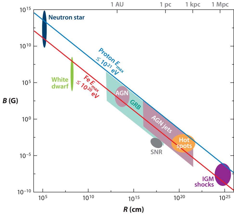
図 1.3 候補天体の大きさと磁場強度を比較した Hillas 図。Kotera and Olinto (2011) の Fig. 8 より引用 [25]。
