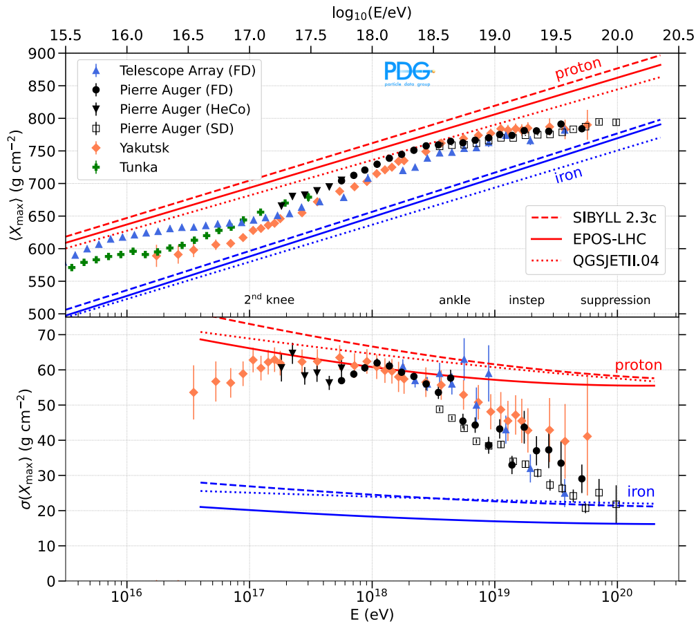
図 1.6 \langle X_{\max} \rangle と \sigma(X_{\max}) のエネルギー依存。PDG のレビュー Cosmic Rays の Fig. 30.8 より引用 [1]。
