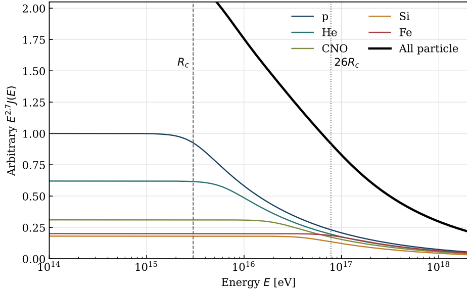
図 1.4 剛性に比例する折れ曲がりを仮定した Peters cycle の模式図。 R_c = 3 \text{ PV} 、 \gamma = 2.70 、 \Delta\gamma = 0.45 とし、元素群の規格化は説明のために選んだ。実験データへのフィットではない [27, 28]。
