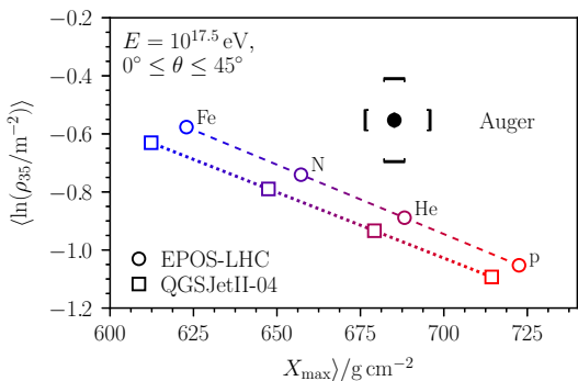
(a) E = 10^{17.5} \text{ eV}
