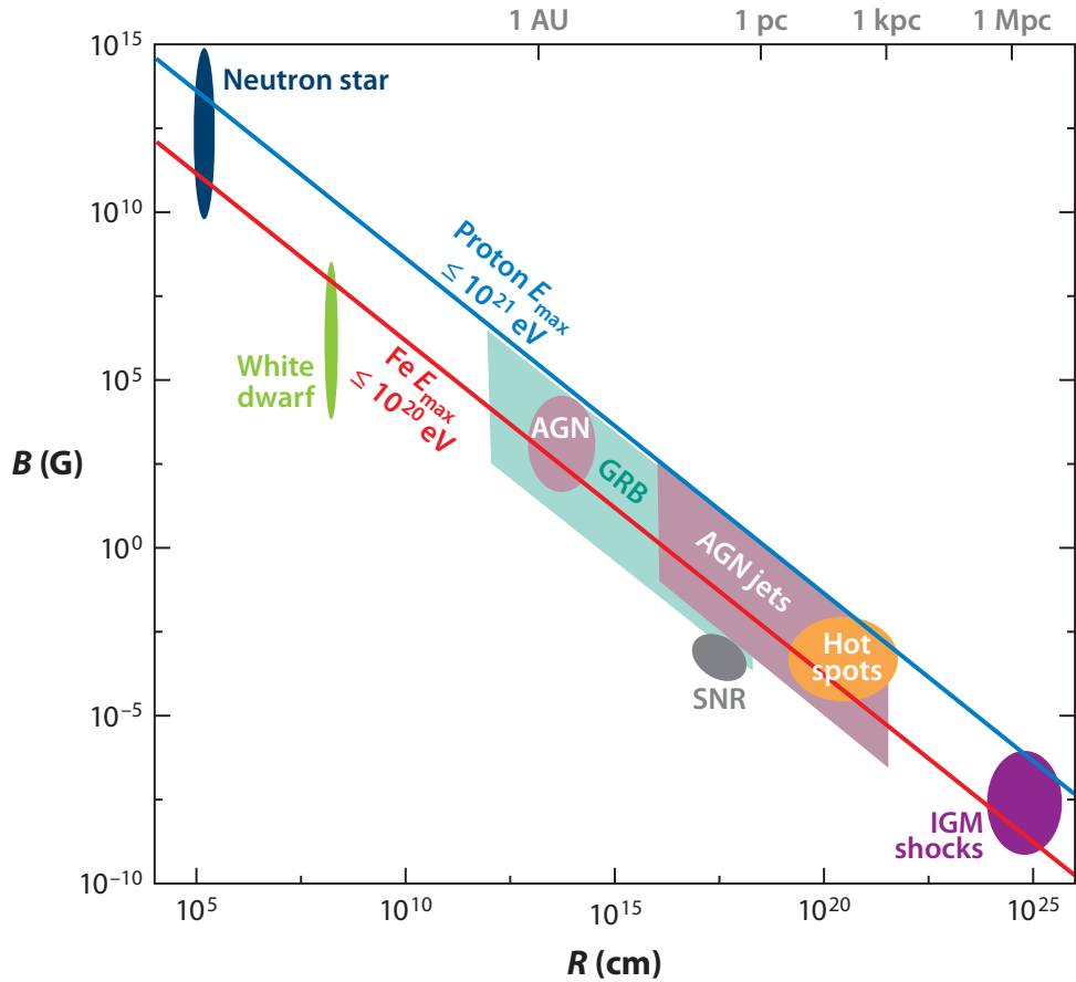
図 1.4 候補天体の大きさと磁場強度を比較した Hillas 図。Kotera and Olinto (2011) の Fig. 8 より引用 [33]。
