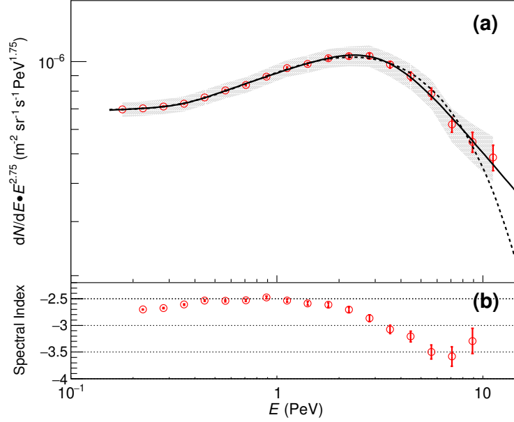
図 1.6 LHAASO が測定した陽子エネルギースペクトル（上）と局所スペクトル指数（下）。赤点は測定値、灰色帯は系統的な不確かさを表す。実線は 3 つのべき乗則成分による適合、破線は 2 つのべき乗則成分と指数関数的カットオフによる適合である。LHAASO Collaboration (2025) の Fig. 2 より引用 [43]。
