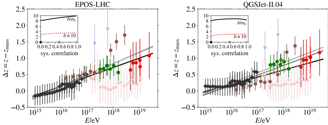
図 2.2 8 つの空気シャワー実験によるミュオン測定を共通尺度で比較したメタ解析。縦軸は質量組成の期待値を差し引いた \Delta z = z - z_{\text{mass}} 、横軸は一次エネルギーである。左は EPOS-LHC、右は QGSJetII-04 に対する比較を示す。直線は実験内の系統的な不確かさの相関を変えた適合であり、KASCADE-Grande と EAS-MSU の点はエネルギースケールを相互較正していない。Dembinski et al. (2019) の Fig. 10 より引用 [69]。
