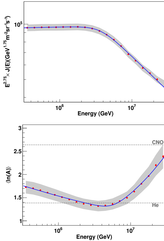
図 1.5 LHAASO-KM2A が測定した全粒子エネルギースペクトル（上）と質量数の対数の平均 \langle \ln A \rangle （下）。灰色帯は系統的不確かさ、青線は折れ曲がりを含む適合結果を表す。LHAASO Collaboration (2024) の Fig. 3 より引用 [13]。
