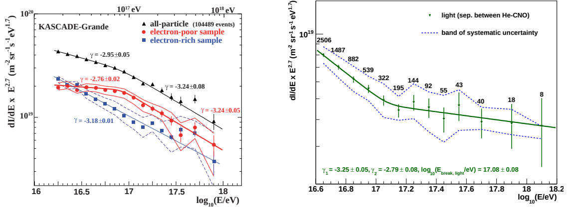
図 1.8 KASCADE-Grande が再構成した質量群別エネルギースペクトル。左は全粒子、電子に乏しい質量群、電子に富む質量群の比較であり、電子に乏しい質量群は約 8 \times 10^{16} eV で急峻化する。右では、電子に富む質量群のスペクトルの傾きが約 10^{17.08} eV から緩やかになる。左は KASCADE-Grande Collaboration (2011) の Fig. 4、右は同 Collaboration (2013) の Fig. 5 より引用 [45, 49]。
