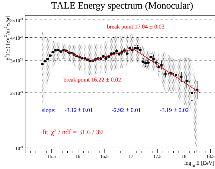
図 1.9 TALE 単眼解析による 2 PeV から 2 EeV の全粒子エネルギースペクトル。赤線は折れ曲がりを含む適合、灰色帯は系統的な不確かさを表す。TALE Collaboration (2018) の Fig. 20 より引用 [14]。
