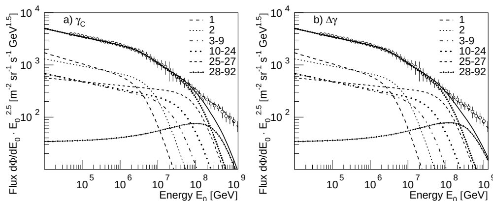
図 1.7 リジディティ依存のカットオフを仮定した poly-gonato モデルによる全粒子スペクトルと質量群別の寄与。左は全質量群でカットオフ後の指数 \gamma_c を共通とした場合、右は指数変化 \Delta\gamma を共通とした場合である。凡例の数字は核電荷 Z の範囲を表す。Hörandel (2003) の Fig. 11 より引用 [36]。
