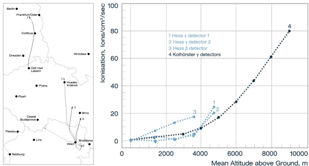
図 1.1 Hess が 1912 年に実施した 7 回の気球飛行経路 (左)。右は、Hess の第 7 回飛行と Kolhörster による飛行で測定した電離率を高度に対して示す。地上で測定した電離率は差し引かれている。De Angelis and Arcaro b. Schultz (2018) の Fig. 3 より引用 [4]。
