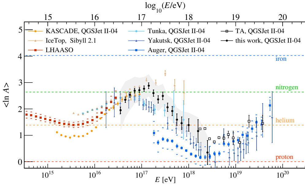
図 1.3 宇宙線の質量数の対数の平均 \langle \ln A \rangle 。TALE ハイブリッド質量組成測定 of Fig. 22 より引用 [21]。
