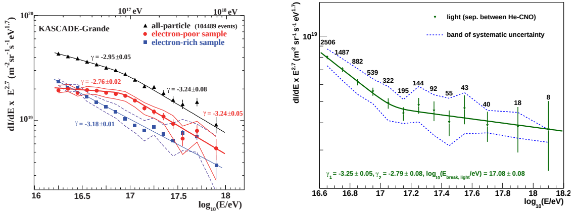
図 1.8 KASCADE-Grande が再構成した質量群別エネルギースペクトル。左は全粒子、電子に乏しい重成分、電子に富む軽成分の比較であり、重成分は約 8 \times 10^{16} eV で急峻化する。右は軽成分スペクトルであり、約 10^{17.08} eV に硬化が見られる。左は KASCADE-Grande Collaboration (2011) の Fig. 4、右は同 Collaboration (2013) の Fig. 5 より引用 [43, 47]。
