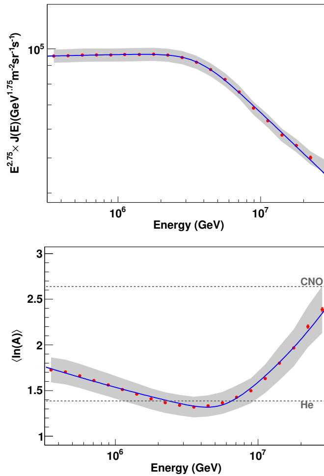
図 1.5 LHAASO-KM2A が測定した全粒子エネルギースペクトル（上）と平均対数質量 \langle \ln A \rangle （下）。灰色帯は系統的不確かさ、青線は折れ曲がりを含む適合結果を表す。LHAASO Collaboration (2024) の Fig. 3 より引用 [11]。
