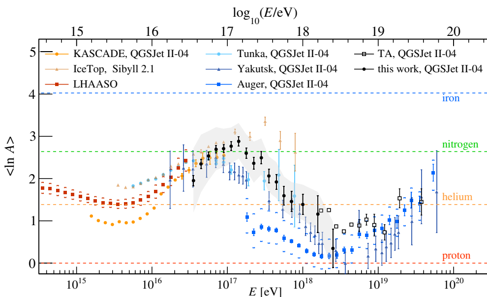
図 1.3 宇宙線の平均対数質量 \langle \ln A \rangle 。TALE ハイブリッド質量組成測定 Fig. 22 より引用 [19]。
