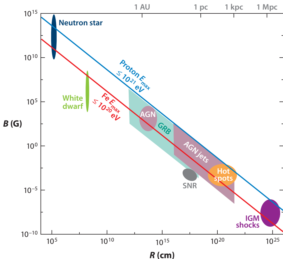
図 1.4 候補天体の大きさと磁場強度を比較した Hillas 図。Kotera and Olinto (2011) の Fig. 8 より引用 [31]。
