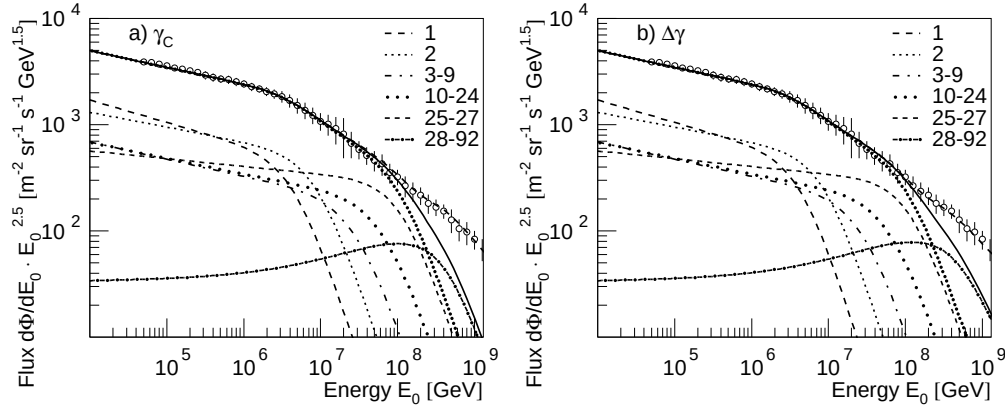
図 1.7 剛性依存カットオフを仮定した poly-gonato モデルによる全粒子スペクトルと元素群別寄与。左は全元素群でカットオフ後の指数 \gamma_c を共通とした場合、右は指数変化 \Delta\gamma を共通とした場合である。凡例の数字は核電荷 Z の範囲を表す。Hörandel (2003) の Fig. 11 より引用 [34]。
