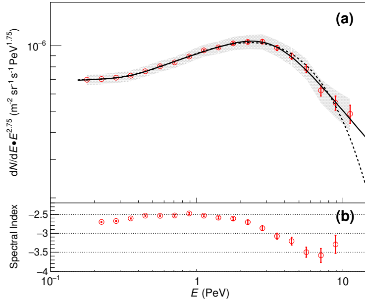
図 1.6 LHAASO が測定した陽子エネルギースペクトル（上）と局所冪指数（下）。赤点は測定値、灰色帯は系統的な不確かさを表す。実線は三つの冪則成分による適合、破線は二つの冪則成分と指数関数的カットオフによる適合である。LHAASO Collaboration (2025) の Fig. 2 より引用 [41]。
