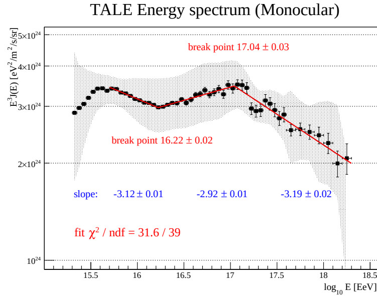
図 1.9 TALE 単眼解析による 2 PeV から 2 EeV の全粒子エネルギースペクトル。赤線は折れ曲がりを含む適合、灰色帯は系統的な不確かさを表す。TALE Collaboration (2018) の Fig. 20 より引用 [12]。
