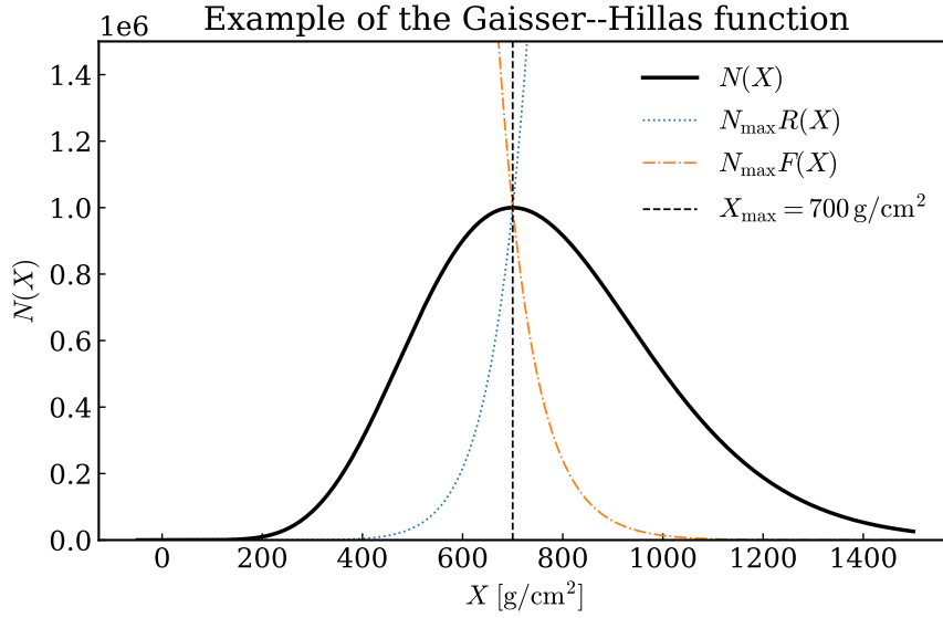
図 2.2 Gaisser–Hillas 関数の例。 N_{\max} = 10^6 、 X_{\max} = 700 \text{ g/cm}^2 、 X_0^{\text{GH}} = -50 \text{ g/cm}^2 、 \Lambda = 70 \text{ g/cm}^2 とした。
