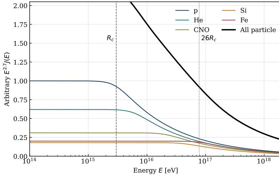
図 1.4 剛性に比例する折れ曲がり仮定した Peters cycle の模式図。 R_c = 3 PV、 \gamma = 2.70 、 \Delta\gamma = 0.45 とし、元素群の規格化は説明のために選んだ。LHAASO を含む個別実験データへのフィットではない [36, 37]。
