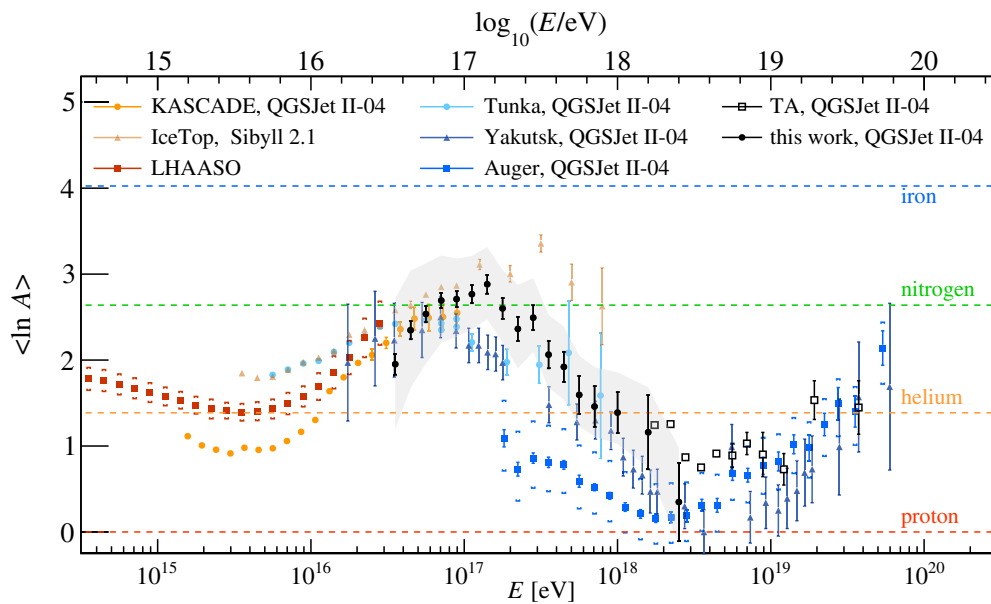
図 1.5 宇宙線の平均対数質量 \langle \ln A \rangle 。TALE ハイブリッド質量組成測定 Fig. 22 より引用 [56]。
