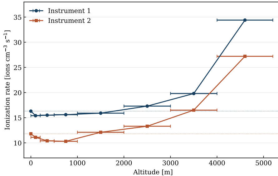
図 1.1 Hess の気球実験で得られた高度区間別の平均電離率。横方向の誤差棒は測定値の統計誤差ではなく、原論文の高度区間を表す。Hess (1912) の平均値表に基づいて本稿で作成した [4, 5]。
