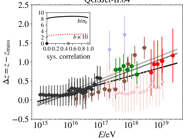
QGSJet-II.04
