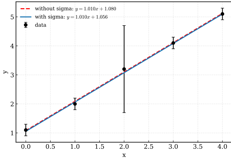
図 10.1 sigma の有無によるフィット結果の違い。不確かさが点ごとに異なる場合、 sigma の指定によって各残差の寄与が変わる。
