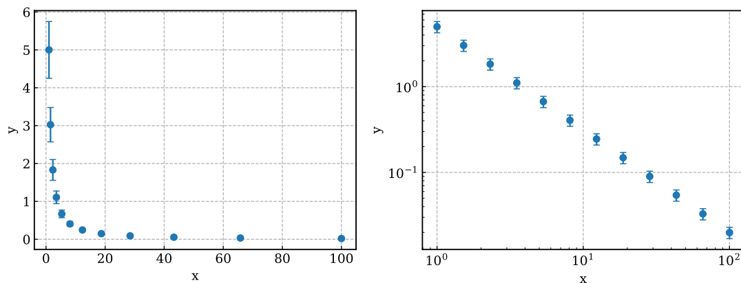
図 9.11 エラーバーと対数軸の設定例。左は線形軸、右は x 軸と y 軸の両方を対数尺度にした図。
