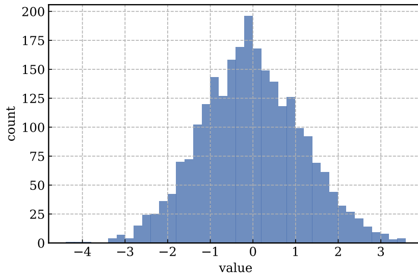
図 9.1 入力配列 values を 40 ビンへ数え上げたヒストグラム。横軸は値、縦軸は各ビンに含まれる要素数を表す。
