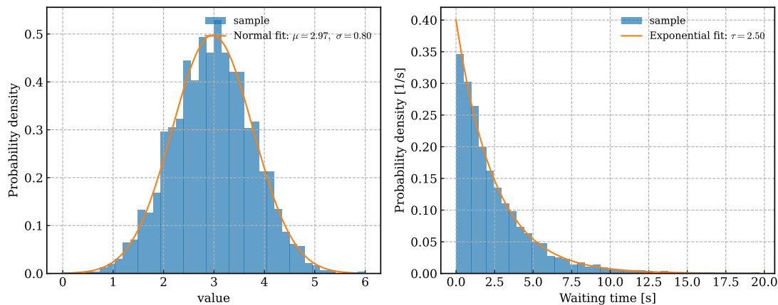
図 9.12 Matplotlib による分布図とフィットの例。左はガウシアン型、右は指数分布であり、どちらもヒストグラムの上にフィット曲線を重ね、凡例に分布名と推定パラメータを示している。
