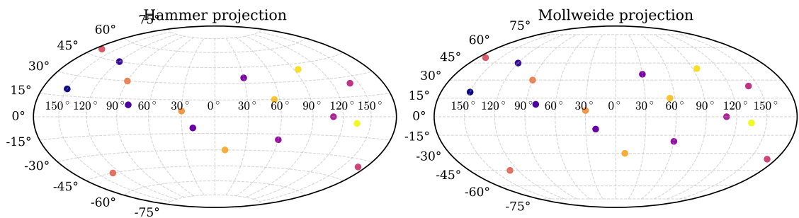
図 9.5 Hammer 図法と Mollweide 図法の例。どちらも経度の全範囲と両極を一つの楕円領域内に投影する。
