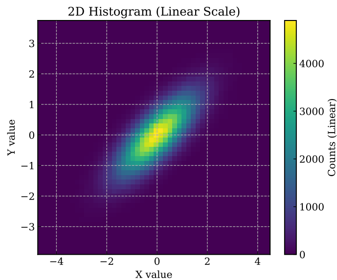
図 9.7 線形カラスケールを用いた 2次元ヒストグラム。中心部の高密度領域に色範囲の大半が割り当てられ、低密度領域の差を識別しにくい。
