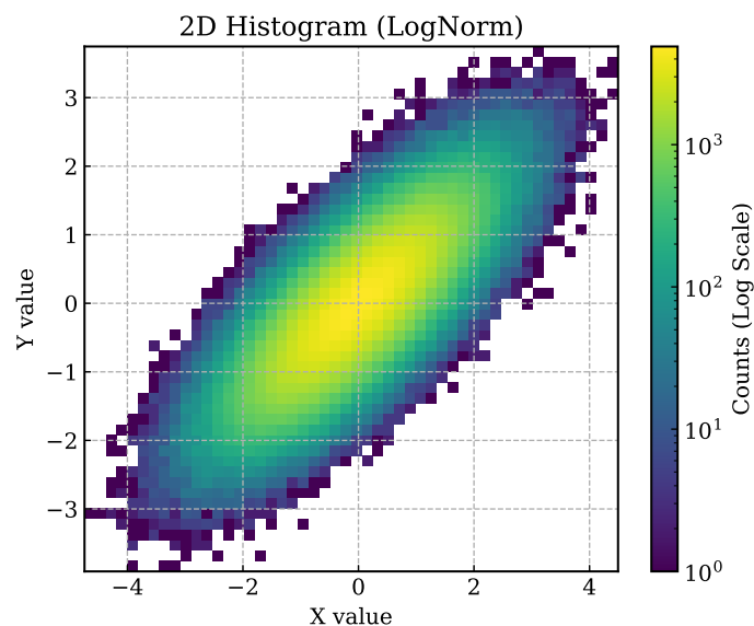
図 9.8 LogNorm を用いた 2 次元ヒストグラム。中心の高密度領域と周囲の低密度領域を同じ色尺度で表す。
