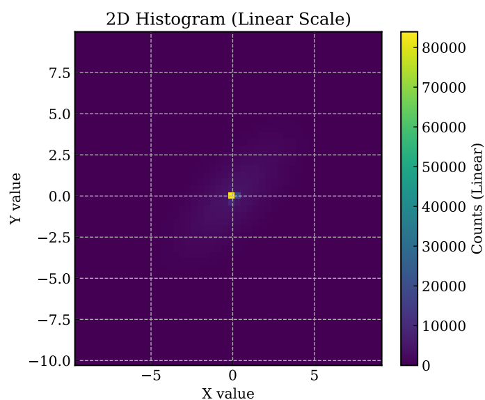
図 9.7 線形カースケールを用いた 2 次元ヒストグラム。中心部の高密度領域に色範囲の大半が割り当てられ、低密度領域の差を識別しにくい。
