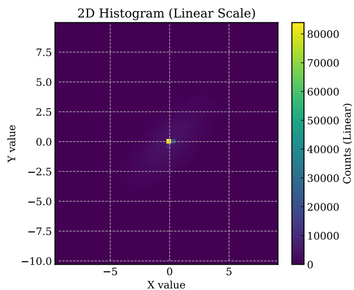
図 9.7 線形カラースケールを用いた 2 次元ヒストグラム。中心部の高密度領域に色範囲の大半が割り当てられ、低密度領域の差を識別しにくい。
