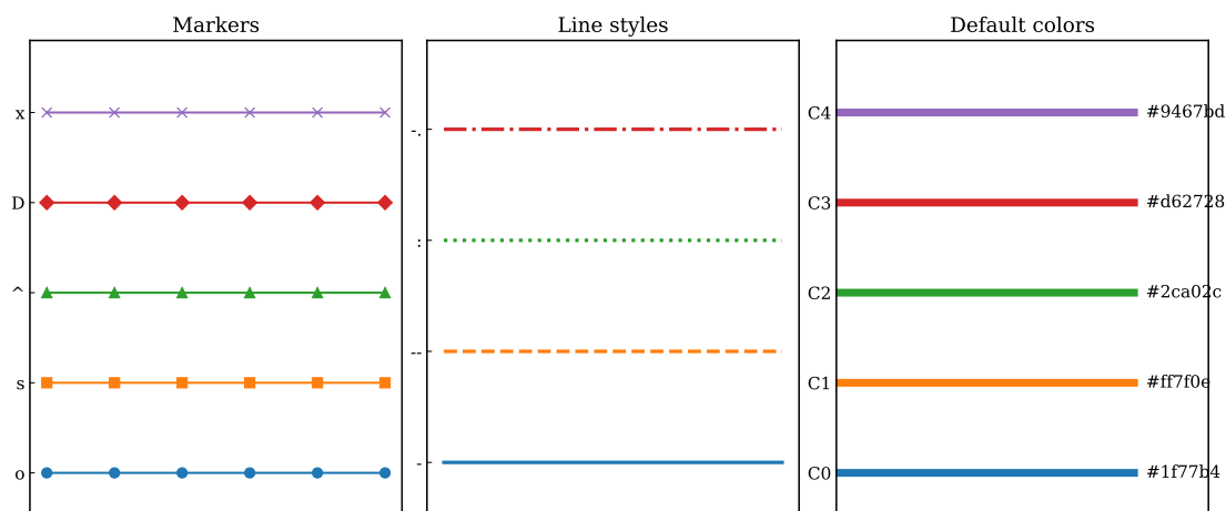
図 9.14 マーカー、線種、既定色の代表例。各指定と描画結果の対応を示す。
