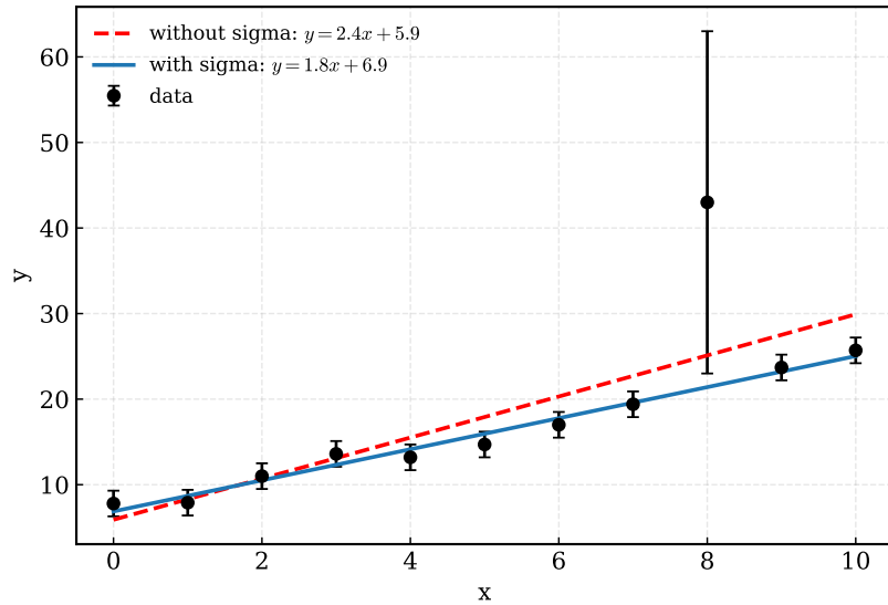
図 10.1 sigma の有無によるフィット結果の違い。誤差の大きい点を適切に弱く扱わないと、結果全体が不安定になる。
