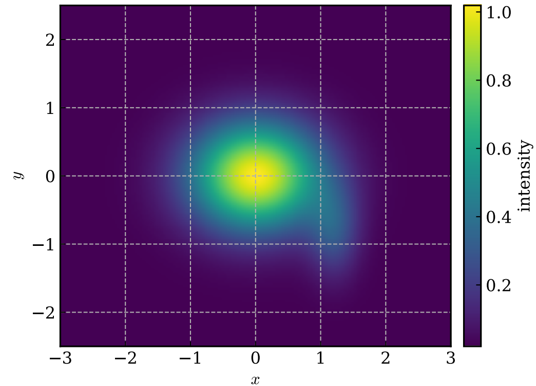
imshow + colorbar
