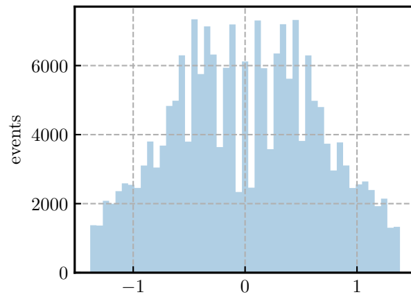
abs_dt_usec
