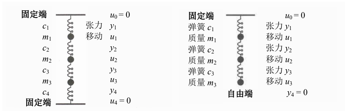
图 10.4: 弹簧线与质量：固定-固定与固定-自由端
