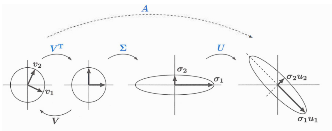
图 7.5: U 与 V 是旋转与可能的反射。 \Sigma 把圆拉伸成椭圆。
