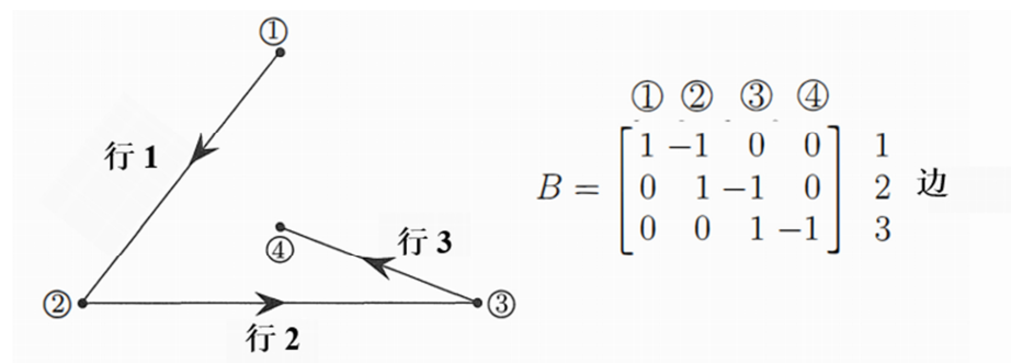
图 10.1*: 3 个边与 4 个节与没有回圈的树，则 B 有独立的行。
