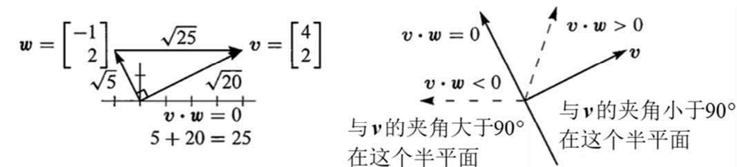
图 1.8: 垂直向量有 \mathbf{v} \cdot \mathbf{w} = 0 ，则 \|\mathbf{v}\|^2 + \|\mathbf{w}\|^2 = \|\mathbf{v} - \mathbf{w}\|^2
