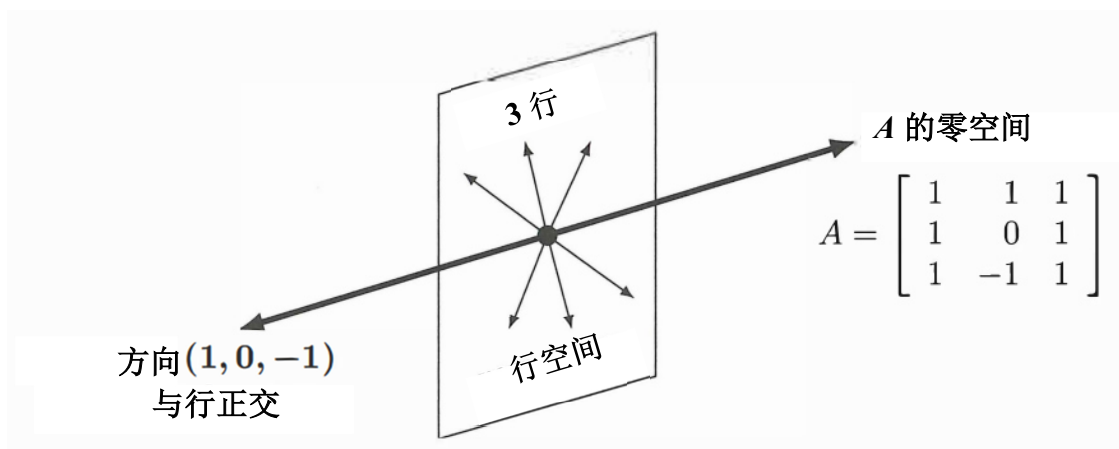
图 4.4: A 的行空间 = 平面, 零空间 = 正交直线, 维度 2 + 1 = 3 。
