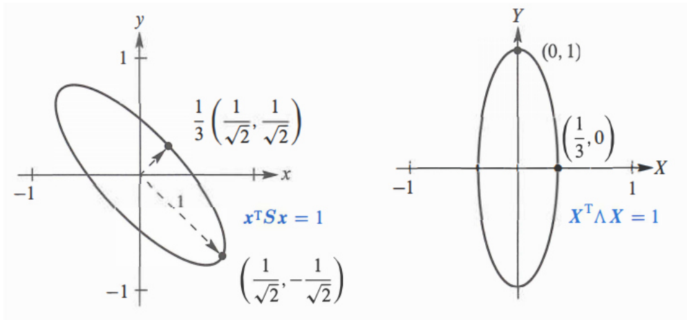
图 6.7: 标题椭圆 5x^2 + 8xy + 5y^2 = 1 , 对齐后是 9X^2 + Y^2 = 1 。
