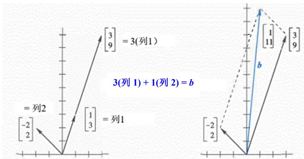
图 2.2: 列图: 列的组合产生右侧的(1, 11)。
