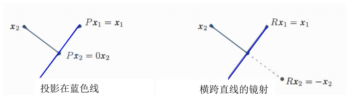
图 6.2: 投影 P 有特征值 1 与 0, 镜射 R 有特征值 \lambda = 1 与 -1。典型的 \mathbf{x} 改变方向, 但是特征向量保持沿着同一直线。
