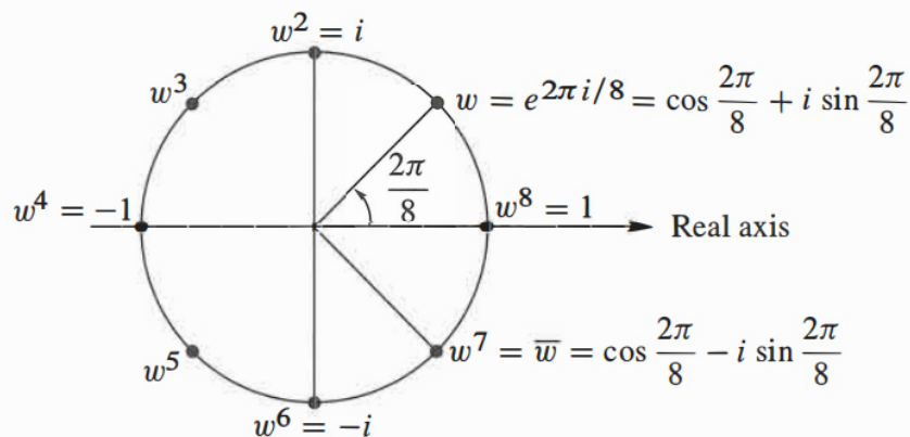
图 9.4: z^8 = 1 的 8 个解是 1, w, w^2, \dots, w^7 ，其中 w = (1+i)/\sqrt{2} 。
