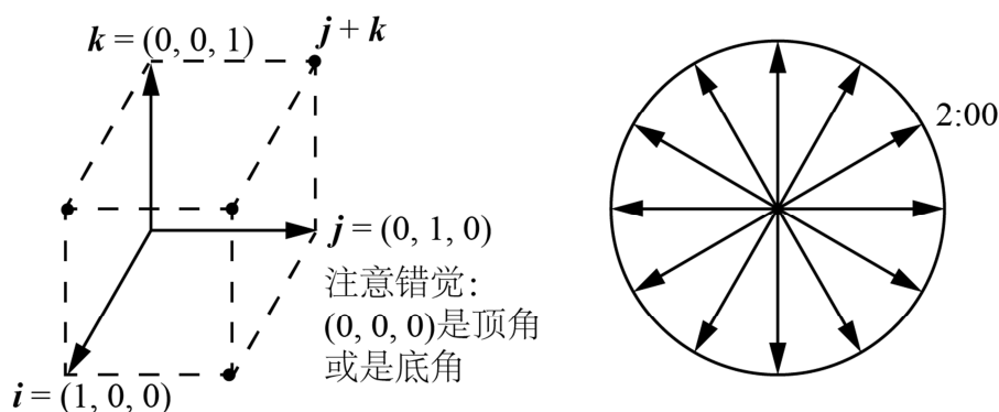
图 1.4: i, j, k 构成的单位立方体与 12 个时钟向量
