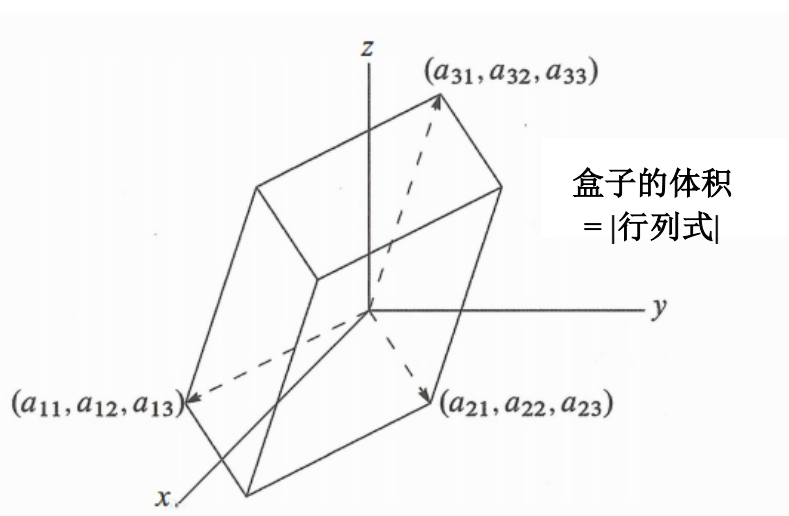
图 5.4: 来自 A 的三个行形成的三维盒子。
