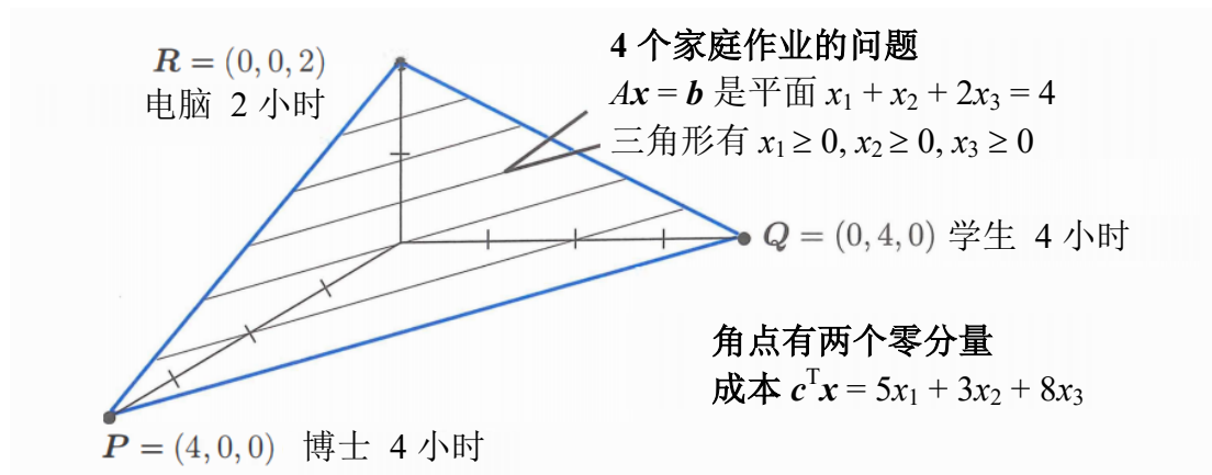
图 10.5: 三角形包含所有非负解: Ax = b 且 x \geq 0 。最低成本解 x^* 是可行集中的角点 P, Q, R 的其中之一。
