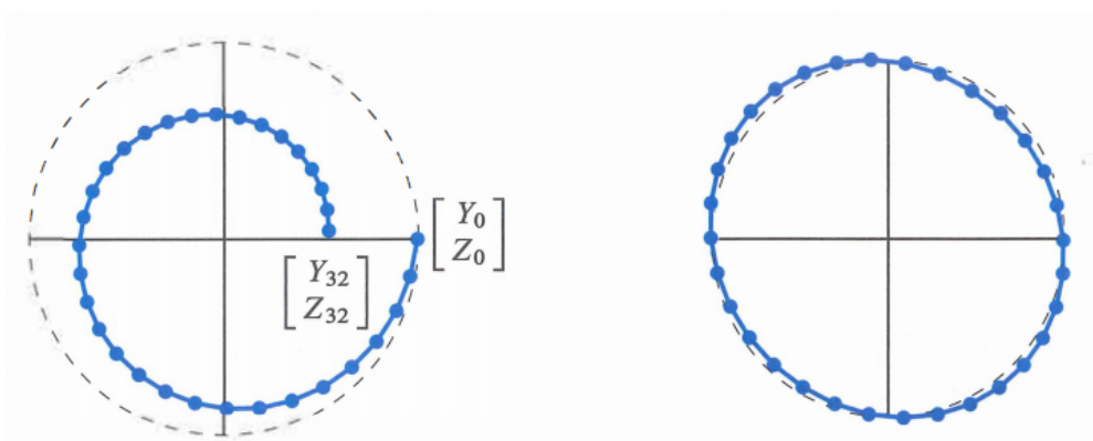
图 6.4: 反向差分螺旋往内，跳背维持与正确圆接近
