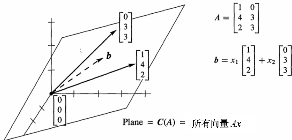
图 3.2: 列空间 C(A) 是一个包含两个列的平面, 当 b 落在这个平面时, Ax = b 有解, 此时 b 是列的组合。
