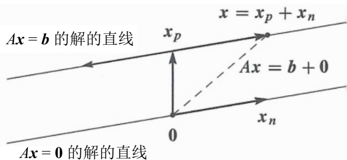
图 3.3: 完整解 = 一个特解 + 所有的零空间解
