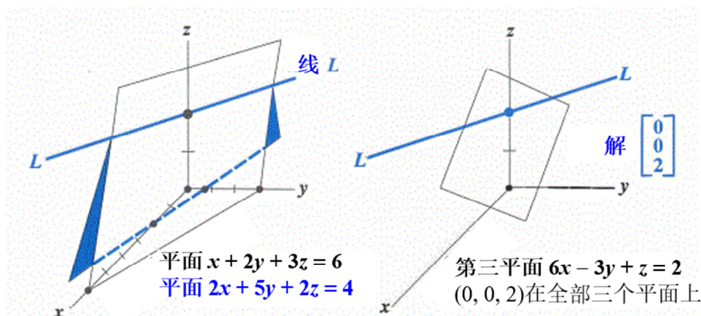
图 2.3：行图：两个平面交于直线 L ，三个平面交于一点
