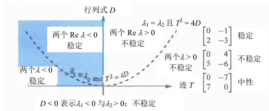
图 6.5: 当迹 < 0 与 \det > 0 , 2 \times 2 矩阵稳定 ( u(t) \rightarrow 0 )
