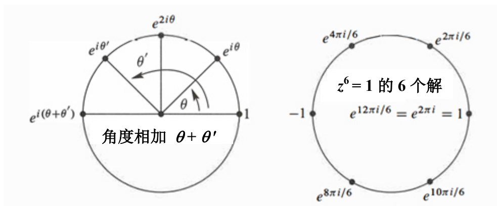
图 9.2: (a) e^{i\theta} 乘 e^{i\theta'} 是 e^{i(\theta+\theta')} (b) e^{2\pi i/n} 的 n 次方是 e^{2\pi i} = 1 。
