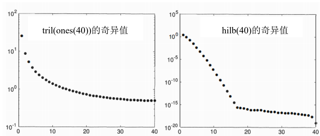
图 7.1: 范例 3-4 中三角 1 矩阵的奇异值(不可压缩)与段落 8.3 的邪恶希尔伯特矩阵 H(i, j) = (i + j - 1)^{-1} : 压缩后使用。
