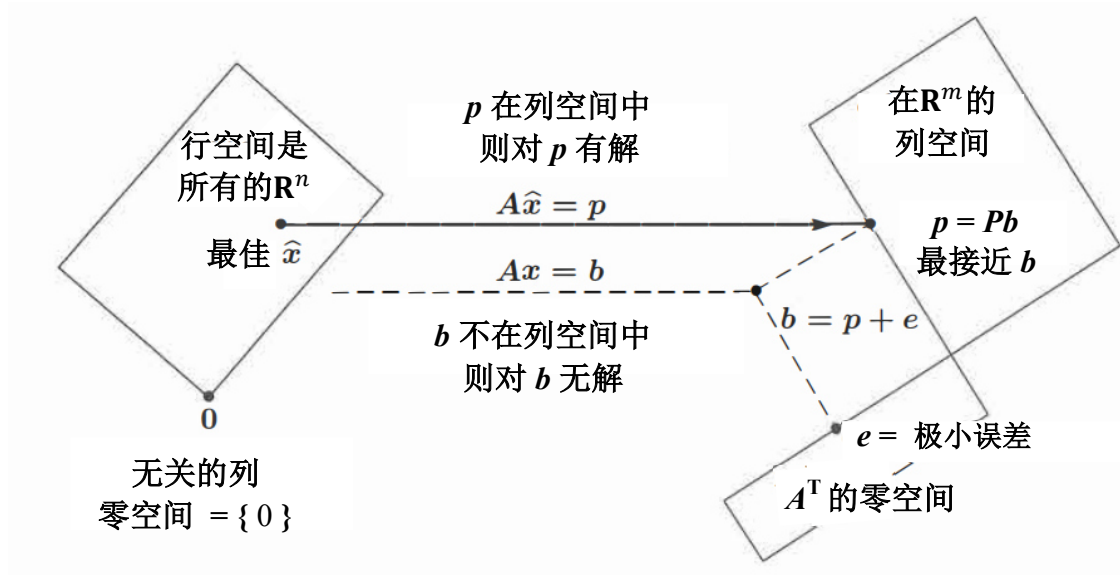
图 4.7: 投影 p = A\hat{x} 接近 b , 所以 \hat{x} 小化 E = \|Ax - b\|^2 。
