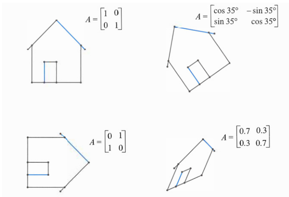
图 8.2: 一间房子的线性变换，利用 plot2d(A*H) 作图。
