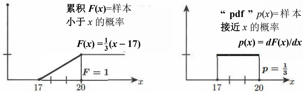
图 12.1: F(x) 是累积分布而且它的导数 p(x) = dF(x)/dx 是概率密度函数(pdf)。对于均匀分布, p(x) 在 17 到 20 之间是常数, p(x) 图形下的总面积是总概率 F = 1 。
