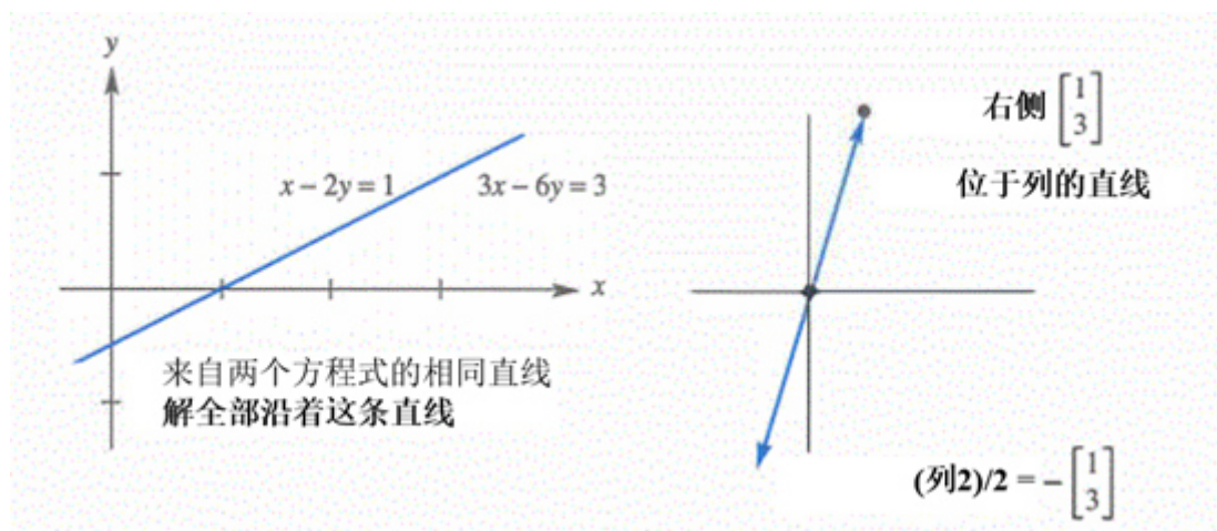
图 2.7: 范例 2 的行图与列图: 无限多解。
