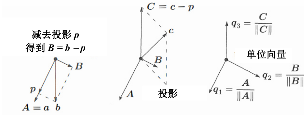
图 4.11: 首先把 b 投影在通过 a 的直线, 求出正交 B 是 b-p 。把 c 投影在 AB 平面, 求出 C=c-p 。除以 \|A\|, \|B\|, \|C\| 。
