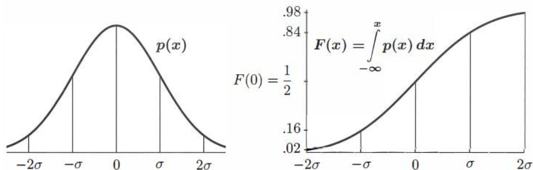
图 12.2: 标准正态分布 p(x) 有平均值 m = 0 与 \sigma = 1 。
