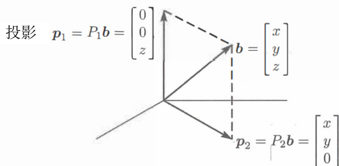
图 4.5: 在 z 轴与 xy 平面的投影 p_1 = P_1 b 与 p_2 = P_2 b 。
