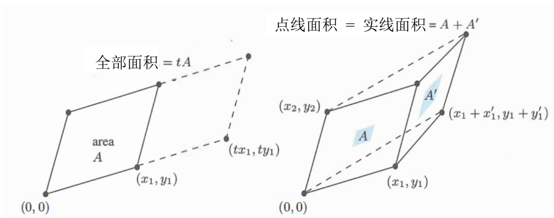
图 5.3: 面积在边 1 遵守线性规则(保持边 (x_2, y_2) 不变)。
