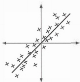
图 7.2: A 中的资料点通常靠近 \mathbf{R}^2 的直线或是 \mathbf{R}^m 的子空间。
