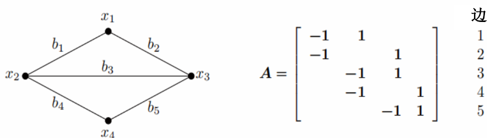
图 3.6: 一个具有 5 个边 4 个节点的“图”, A 是 5 \times 4 的入射矩阵
