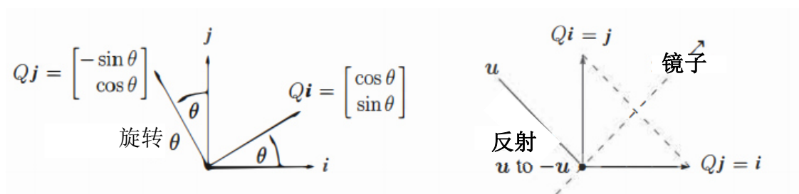
图 4.10: 借由 \mathbf{Q} = \begin{bmatrix} c & -s \\ s & c \end{bmatrix} 旋转以及借由 \mathbf{Q} = \begin{bmatrix} 0 & 1 \\ 1 & 0 \end{bmatrix} 横跨 45^\circ 反射。
