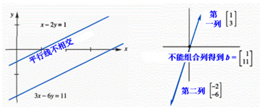
图 2.6: 范例 1 的行图与列图: 无解。
