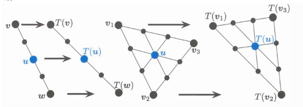
图 8.1：直线到直线，等空间到等空间， u = 0 到 T(u) = 0 。
