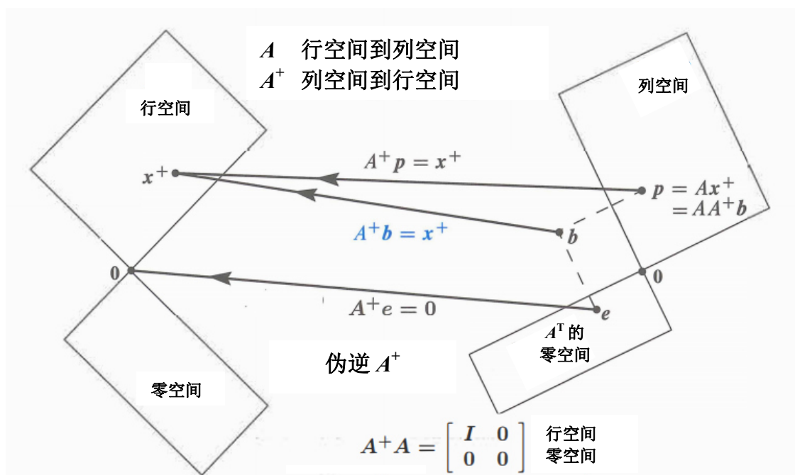
图 7.6: 列空间中的 Ax^+ 回到行空间中的 A^+Ax^+ = x^+ 。
