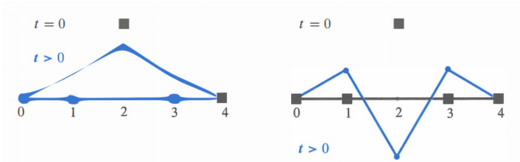
图 6.6: 热从盒子 2 往外扩散(左), 波从盒子 2 传播(右)
