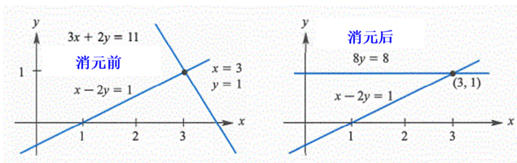
图 2.5：消去 x 使得第二条直线变成水平，则 8y = 8, y = 1 。
