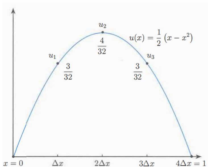
图 10.3: -\frac{d^2u}{dx^2}=1 的解与固定-固定边界 K_0u = (\Delta x)^2f 的解。
