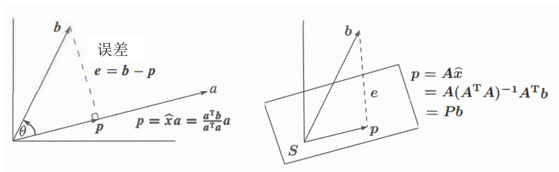
图 4.6: b 在一条直线的投影 p 以及 b 在 S = A 的列空间的投影
