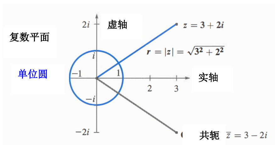
图 9.1: 数字 z = a + bi 对应到点 (a, b) 以及向量 \begin{bmatrix} a \\ b \end{bmatrix} 。
