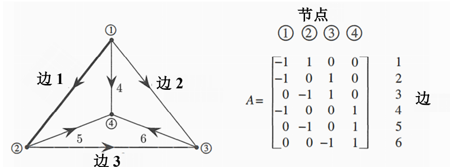
图 10.1: m = 6 个边与 n = 4 个节点的完整图形: 6 \times 4 的关联矩阵 A 。
