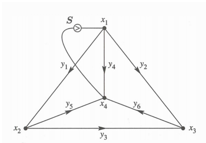
图 10.2: 从节点 4 到 1 有一个电流源 S 的网络电流 y_1 到 y_6 。
