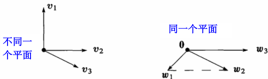
图 3.4: 无关向量 \mathbf{v}_1, \mathbf{v}_2, \mathbf{v}_3 , 只有在 0\mathbf{v}_1 + 0\mathbf{v}_2 + 0\mathbf{v}_3 得到零向量。相关向量 \mathbf{w}_1, \mathbf{w}_2, \mathbf{w}_3 , 组合 \mathbf{w}_1 - \mathbf{w}_2 + \mathbf{w}_3 = (0, 0, 0) 。
