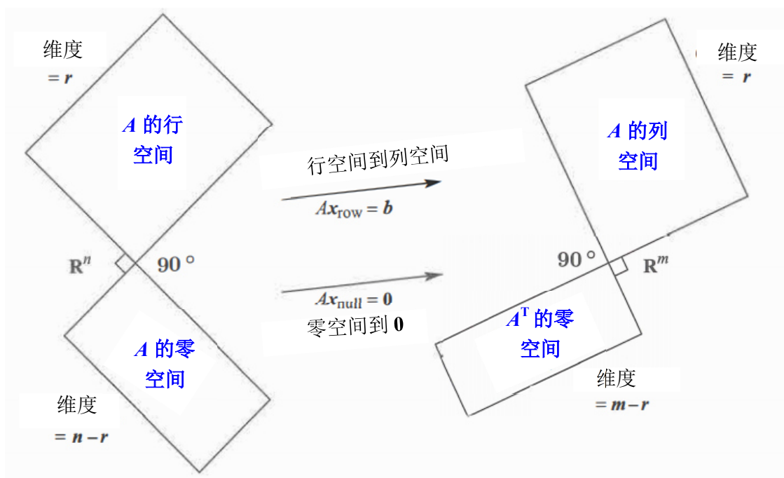
图 4.2: 两对(pairs)正交子空间, 维度总和是 n 与 m 。这是大图——两个子空间在 \mathbf{R}^n 中, 两个子空间在 \mathbf{R}^m 中。
