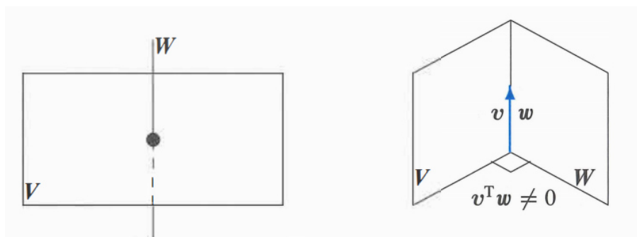
正交平面 V 与直线 W
