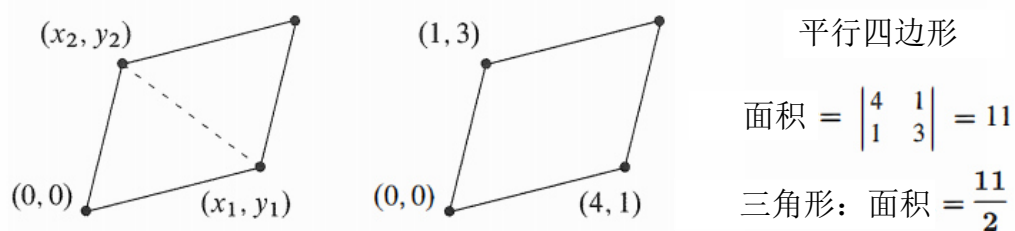
图 5.2: 三角形是平行四边形的一半，面积是行列式的一半。
