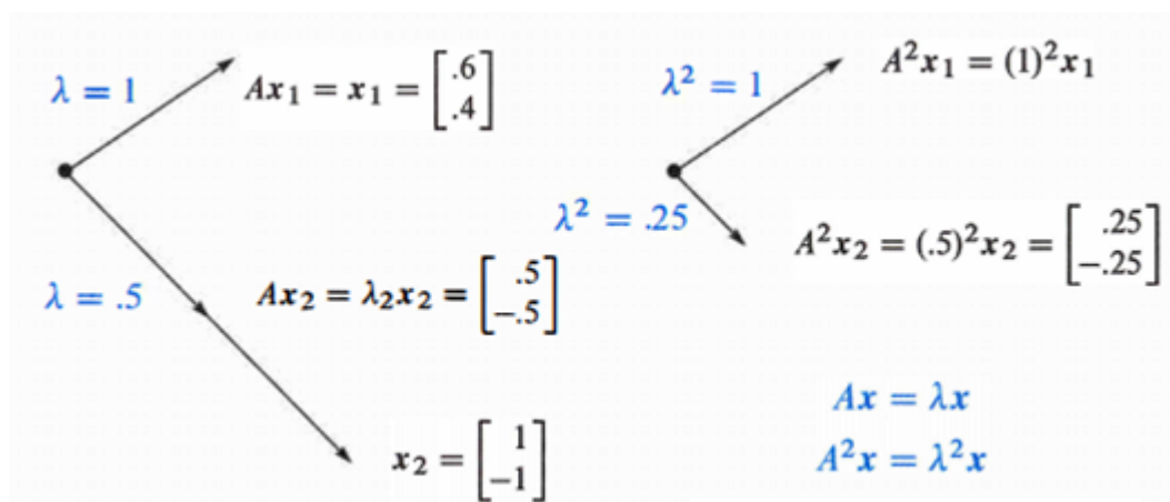
图 6.1: 特征向量维持方向。 A^2\mathbf{x} = \lambda^2\mathbf{x} , 其中 \lambda^2 = 1^2 与 (0.5)^2 。
