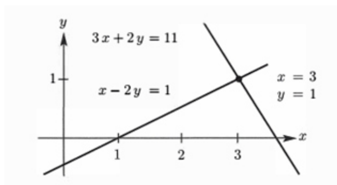
图 2.1：行图：点(3, 1)是两条直线的交点，也是两个方程式的解。
