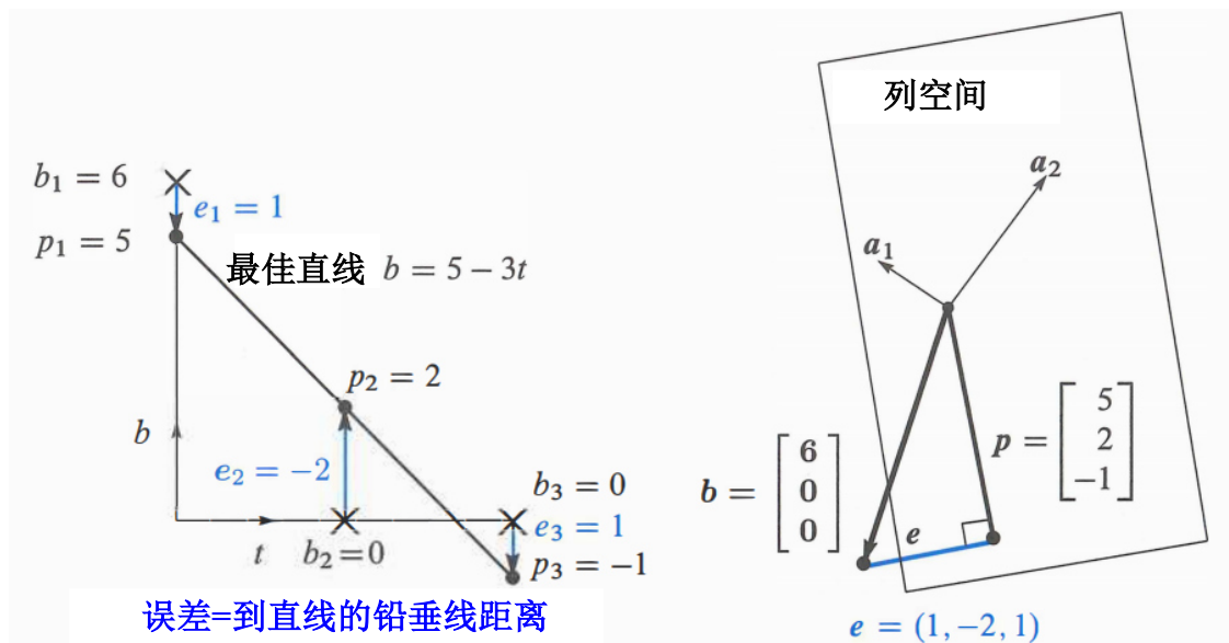
图 4.6: 最佳直线与投影: 两个图形, 同样问题。直线有高度 p = (5, 2, -1) 且误差 e = (1, -2, 1) 。方程式 A^T A \hat{x} = A^T b 得到 \hat{x} = (5, -3) , 相同答案! 最佳直线是 b = 5 - 3t 且最近点是 p = 5a_1 - 3a_2 。
