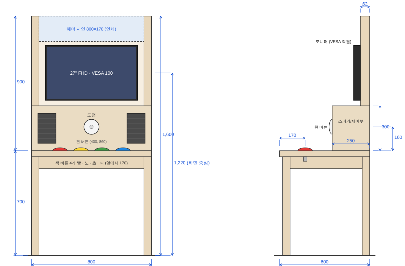
정면 (앞에서). 등판은 뒷다리와 한 몸. 흰 버튼은 하부 박스 앞면.
