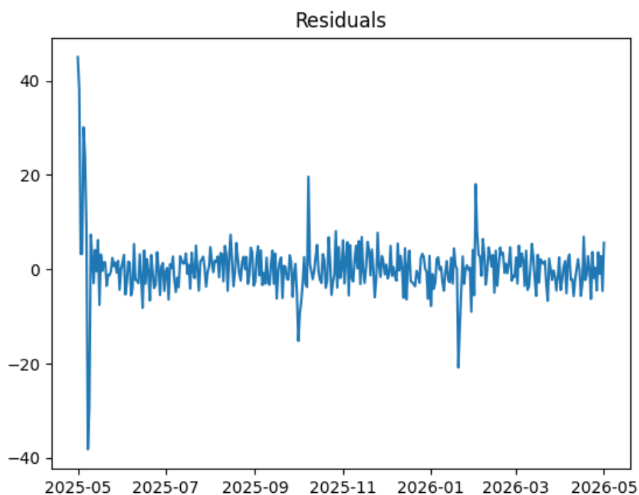
图 6.4 残差序列图
