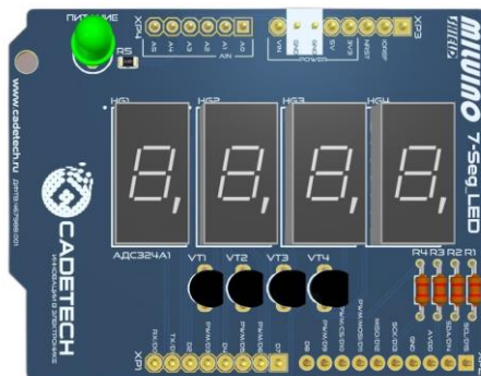
Рисунок 1. – Внешний вид отладочного комплекта для индикатора АЛС324А1 MILUINO SHIELD 7-Seg_LED*
