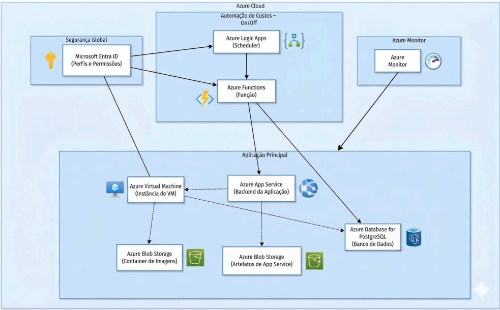
Diagrama de Infraestrutura Azure
