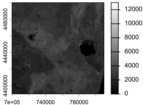
SWIR (B11)
