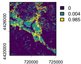
xeric
