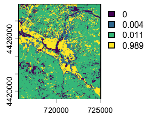
mesic
